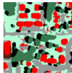
ImageNet + BYOL
