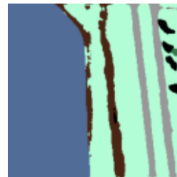
ImageNet + BYOL
