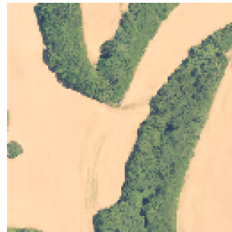
T = 100
