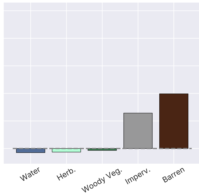
F1 Score
