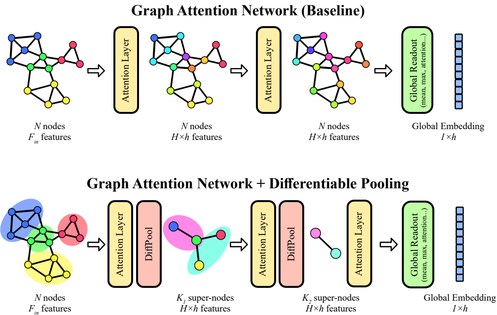
Fig. 3: Comparació visual de les dues arquitectures configurables (una instància de cada branca amb dues capes de processament). Dalt : GAT Baseline, on dues capes d'atenció operen sobre els N nodes originals i un readout global produeix l'embedding final. Baix : GAT+DiffPool amb dos blocs DiffPool ( L_{DP} = 2 , és a dir tres capes GAT intercalades), que col·lapsen progressivament el graf fins a, en aquest cas, dos super-nodes finals.
