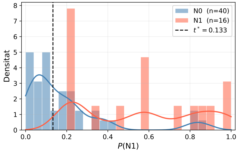
Fig. 9: Distribució de P(N1) sobre el test set (56 pacients) per al model seleccionat GAT Baseline (Grid #1). Blau: N0 ( n=40 ); vermell: N1 ( n=16 ). Línia discontinua: llindar operatiu t^* = 0,133 (tota la distribució N1 queda a la dreta; 23 de 40 N0 queden a l'esquerra).
