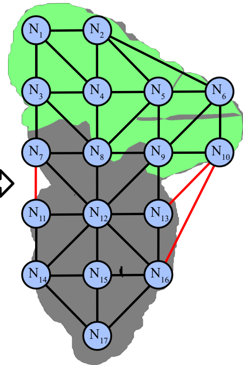
Construcció del graf amb màscara anotada
