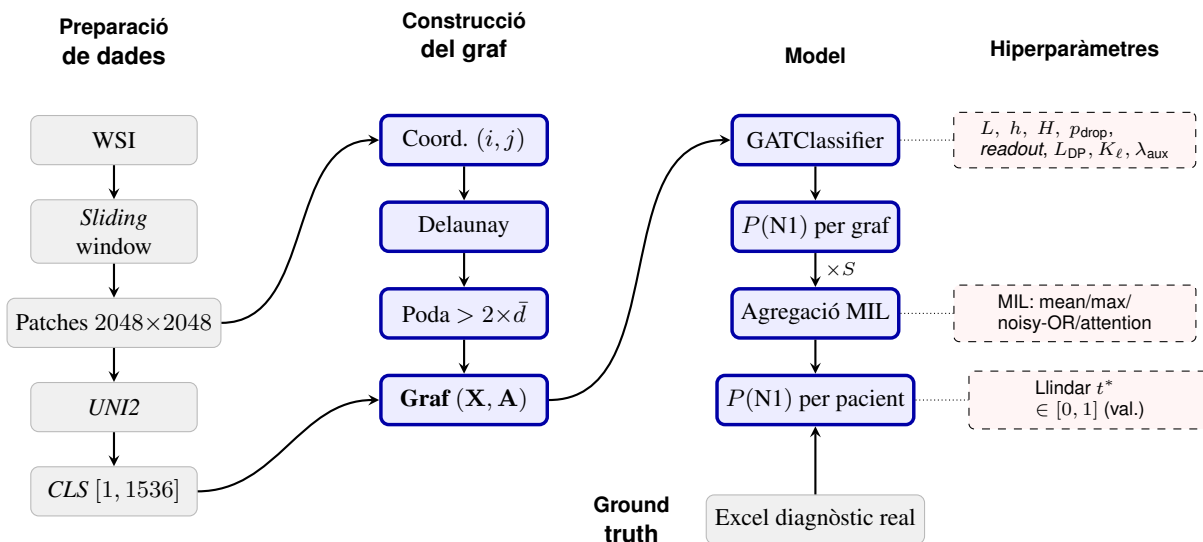
Fig. 7: Diagrama de flux del pipeline complet amb els hiperparàmetres optimitzats (columna dreta, caixes discontinües). Blocs grisos : etapes fetes pels companys de l'equip i dades de referència; blocs blaus : contribucions d'aquest TFG. La fletxa \times S indica que les S seccions d'un pacient es processen com a grafs independents i s'agreguen via MIL per al diagnòstic per pacient.
