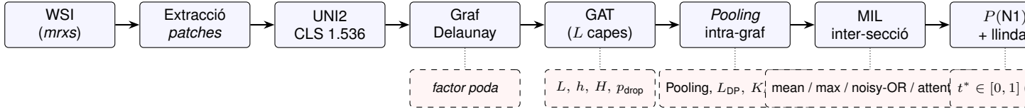
Fig. 3: Pipeline general. Cada bloc representa un mòdul; els hiperparàmetres configurables optimitzats per cerca bayesiana apareixen a sota en línia discontinua. L : nombre de capes GAT; h : dim. oculta; H : nombre de caps d'atenció; L_{DP} : nombre de blocs DiffPool; K_\ell : super-nodes per nivell; \lambda_{aux} : pes del penalty de DiffPool; t^* : llindar de decisió derivat del validation set .
