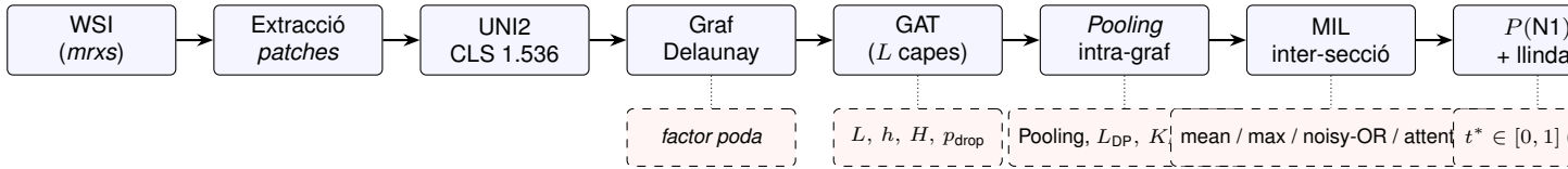
Fig. 3: Pipeline general. Cada bloc representa un mòdul; els hiperparàmetres configurables optimitzats per cerca bayesiana apareixen a sota en línia discontinua. L : nombre de capes GAT; h : dim. oculta; H : nombre de caps d'atenció; L_{DP} : nombre de blocs DiffPool; K_\ell : super-nodes per nivell; \lambda_{aux} : pes del penalty de DiffPool; t^* : llindar de decisió derivat del validation set .
