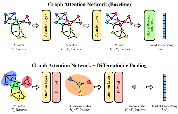
Fig. 4: Comparació visual de les dues arquitectures. Dalt: GAT Baseline, on les capes d'atenció operen sobre els N nodes originals i un readout global produeix l'embedding final. Baix: GAT+DiffPool, on cada capa GAT va seguida d'un bloc DiffPool que col·lapsa progressivament el graf fins als K_{LDP} super-nodes finals, sobre els quals s'aplica un readout global.
