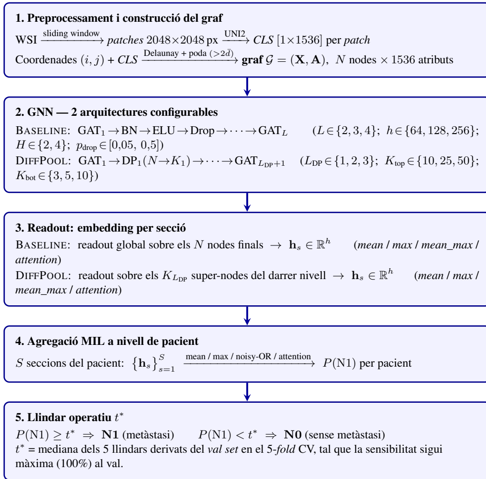
Fig. 8: Diagrama de flux del pipeline complet. Cada bloc és una etapa del procés: (1) preprocessament i construcció del graf a partir de la WSI; (2) processament del graf amb la GNN (dues arquitectures configurables); (3) readout que comprimeix el graf en un vector \mathbf{h}_s per secció; (4) agregació MIL de les S seccions d'un pacient fins a obtenir P(N1) ; (5) decisió binària via el llindar operatiu t^* derivat del val set .
