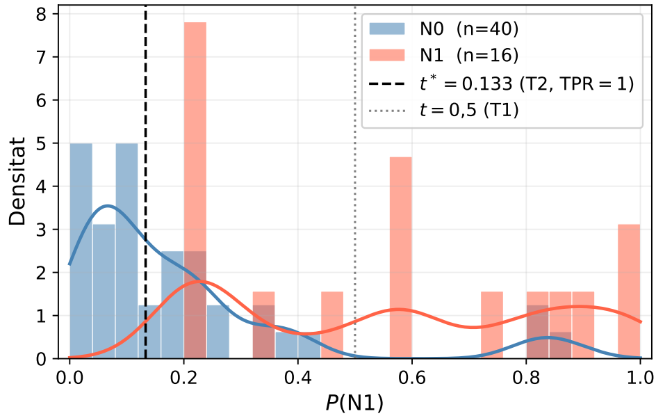
Fig. 10: Distribució de P(N1) sobre el test ( n = 56 ) per al GAT Baseline seleccionat. Blau: N0 ( n = 40 ); vermell: N1 ( n = 16 ). Línia discontínua: t^*=0,133 (T2, TPR= 1); línia puntejada: t=0,5 (T1). Tots els N1 queden a la dreta de t^* .
