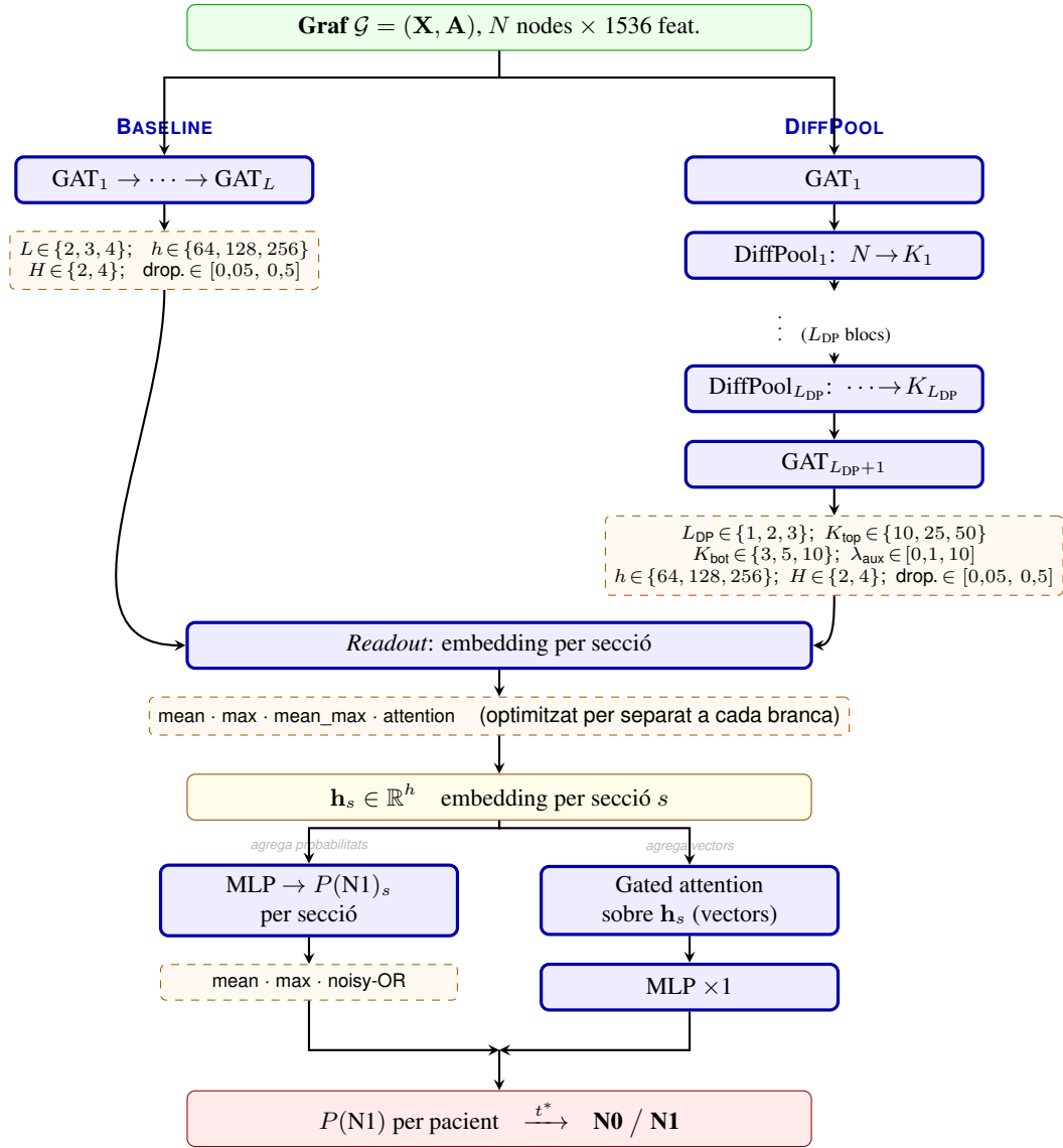
Fig. 9: Variants d'arquitectura del GATClassifier : el mateix graf \mathcal{G} es pot processar per dues branques configurables (BASELINE o DIFFPOOL). Totes dues convergeixen en un readout unificat (caixes portocalles) que produeix l'embedding \mathbf{h}_s \in \mathbb{R}^h per secció; l'opció de readout s'optimitza de forma independent per a cada branca. L'agregació MIL bifurca de nou: mean/max/noisy-OR apliquen el MLP per secció i n'agreguen els escalars ; attention (gated) agrega primer els vectors \mathbf{h}_s amb pesos d'atenció apresos (matrius \mathbf{V}, \mathbf{U} i vector \mathbf{w} [12]) i aplica el MLP una sola vegada sobre l'embedding agregat. L : capes GAT; h : dim. oculta; H : caps d'atenció; L_{DP} : blocs DiffPool; K_\ell : super-nodes per nivell; \lambda_{aux} : pes pèrdua auxiliar DiffPool; t^* : llindar derivat del val set (Secció 6.1).
