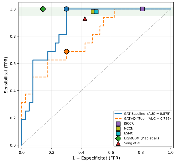
Fig. 4: Corbes ROC al conjunt de test ( n = 56 ) del GAT Baseline (model seleccionat; AUC = 0,875) i del GAT+DiffPool (millor configuració; AUC = 0,786). Els cercles marquen els llindars t^* de cada model (derivats del val set sense data leakage ): t^* = 0,133 per al Baseline (sens. = 100%, espec. = 57,5%) i t^* = 0,303 per al DiffPool (sens. = 62,5%, espec. = 70,0%). Es superposen els punts operatius de JSCCR, NCCN i ESMO (quadrats), LightGBM [21] (diamant) i Song et al. [25] (triangle).
