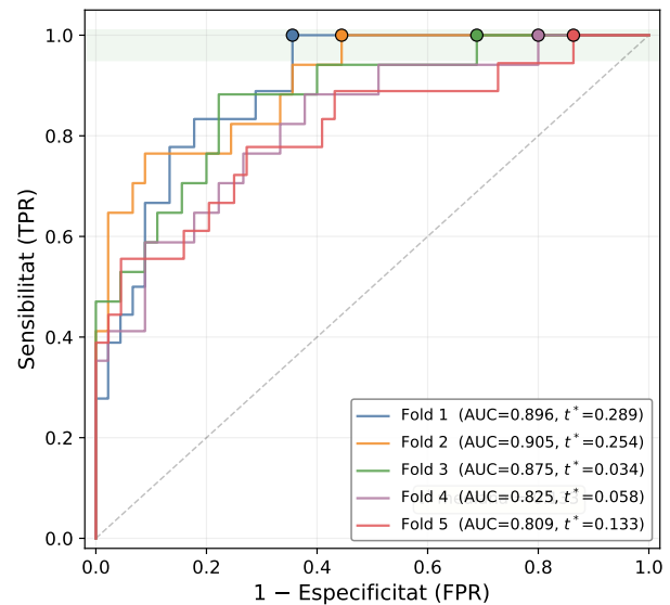
Fig. 5: Corbes ROC dels 5 folds de validació creuada (GAT Baseline). Cada cercle marca el llindar màxim amb TPR = 1 del seu fold ; la mediana dels 5 llindars ( t^* = 0,133 , encadrat groc) s'aplica al test.
