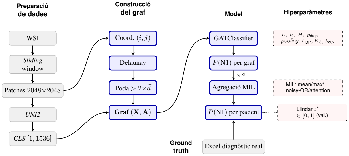
Fig. 6: Diagrama de flux del pipeline complet amb hiperparàmetres optimitzats per la cerca bayesiana (columna dreta, caixes vermelles discontinues). Blocs grisos : etapes realitzades pels companys de l'equip i dades de referència. Blocs blaus : contribucions d'aquest TFG. La fletxa \times S indica que les S seccions d'un pacient es processen com a grafs independents i les P(N1) s'agreguen via MIL per obtenir el diagnòstic per pacient, que es compara amb el diagnòstic real de l'Excel. L : capes GAT; h : dim. oculta; H : caps d'atenció; L_{DP} : blocs DiffPool; K_{\ell} : super-nodes per nivell; \lambda_{aux} : pes del penalty DiffPool; t^* : llindar de decisió derivat del val set.
