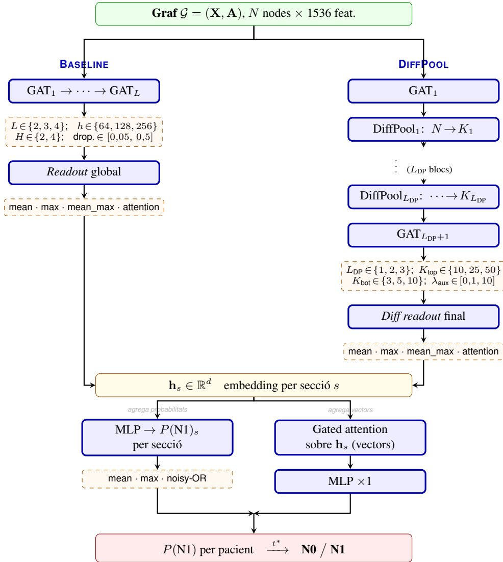
Fig. 7: Variants d'arquitectura del GATClassifier : el mateix graf \mathcal{G} es pot processar per dues branques configurables (BASELINE o DIFFPOOL), cadascuna amb la seva pròpia estratègia de readout intra-secció (caixes taronges discontinües). Totes dues convergeixen en un embedding \mathbf{h}_s per secció. L'agregació MIL bifurca de nou: mean/max/noisy-OR apliquen el MLP per secció per obtenir P(N1)_s i n'agreguen els escalars ; attention (gated) agrega primer els vectors \mathbf{h}_s (amb pesos d'atenció apresos) i aplica el MLP una sola vegada . L : capes GAT; h : dim. oculta; H : caps d'atenció; L_{DP} : blocs DiffPool; K_\ell : super-nodes per nivell; \lambda_{aux} : pes de la pèrdua auxiliar de DiffPool; t^* : llindar derivat del val set (Secció 7.3).
