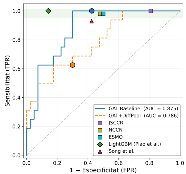
Fig. 5: Corbes ROC al conjunt de test ( n = 56 ) del GAT Baseline (model seleccionat; AUC = 0,875) i del GAT+DiffPool (millor configuració; AUC = 0,786). Els cercles marquen els llindars t^* de cada model (derivats del val set): t^* = 0,133 per al Baseline (sens. = 100%, espec. = 57,5%) i t^* = 0,303 per al DiffPool (sens. = 62,5%, espec. = 70,0%). Es superposen els punts operatius de JSCCR, NCCN i ESMO (quadrats), LightGBM [11] (diamant) i Song et al. [26] (triangle).
