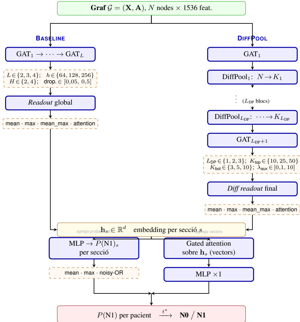
Fig. 7: Variants d'arquitectura del GATClassifier : el mateix graf G es pot processar per dues branques configurables (BASELINE o DIFFPOOL), cadascuna amb la seva pròpia estratègia de readout intra-secció (caixes taronges discontinües). Totes dues convergeixen en un embedding \mathbf{h}_s per secció. L'agregació MIL bifurca de nou: mean/max/noisy-OR apliquen el MLP per secció per obtenir P(N1)_s i n'agreguen els escalars ; attention (gated) agrega primer els vectors \mathbf{h}_s (amb pesos d'atenció apresos) i aplica el MLP una sola vegada . L : capes GAT; h : dim. oculta; H : caps d'atenció; L_{DP} : blocs DiffPool; K_\ell : super-nodes per nivell; \lambda_{aux} : pes de la pèrdua auxiliar de DiffPool; t^* : llindar derivat del val set (Secció 7.3).
