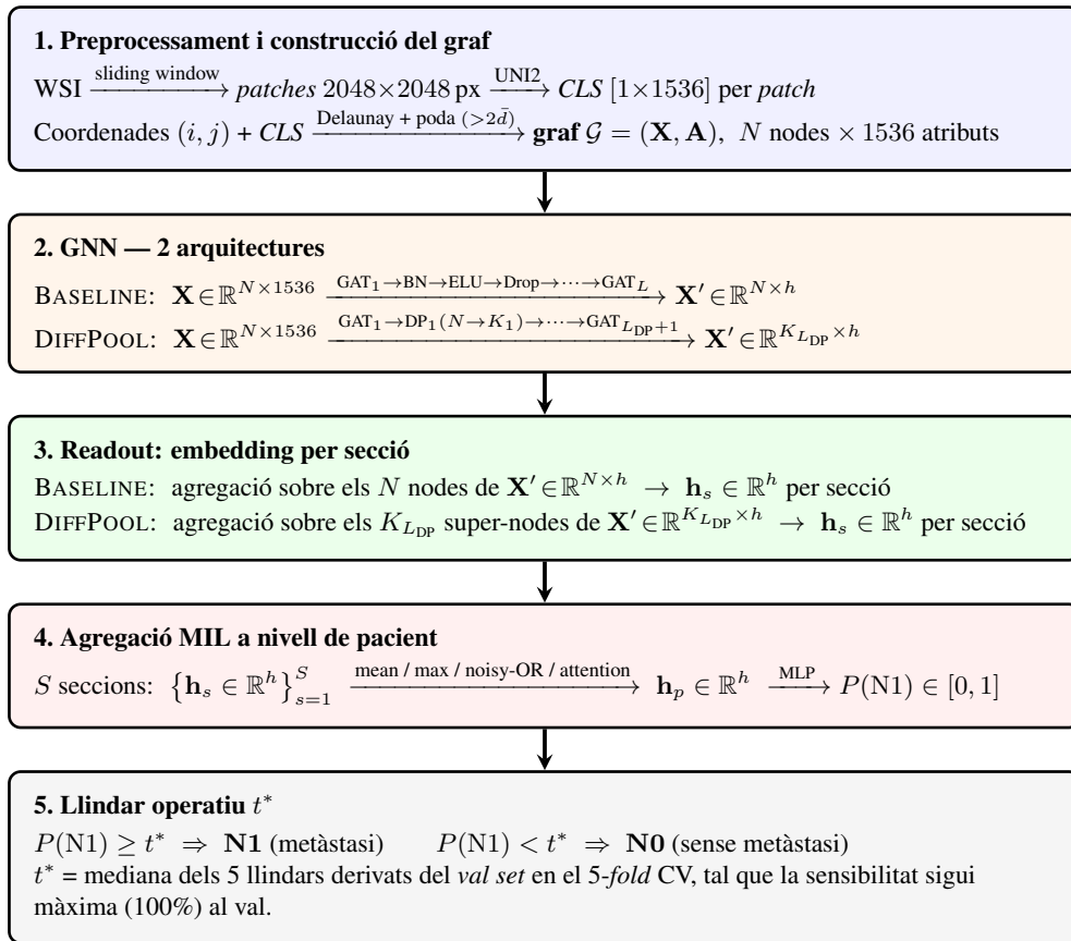
Fig. 8: Diagrama de flux del pipeline complet, de la WSI a la decisió N0/N1. Els cinc blocs es descriuen a la Secció 5.1.
