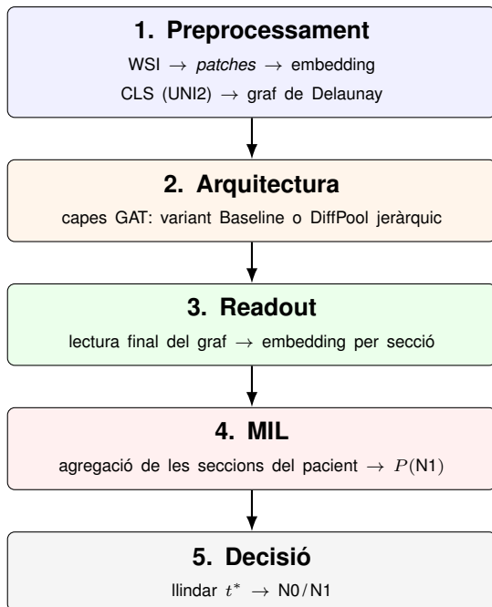
Fig. 2: Visió general del pipeline en cinc blocs.
