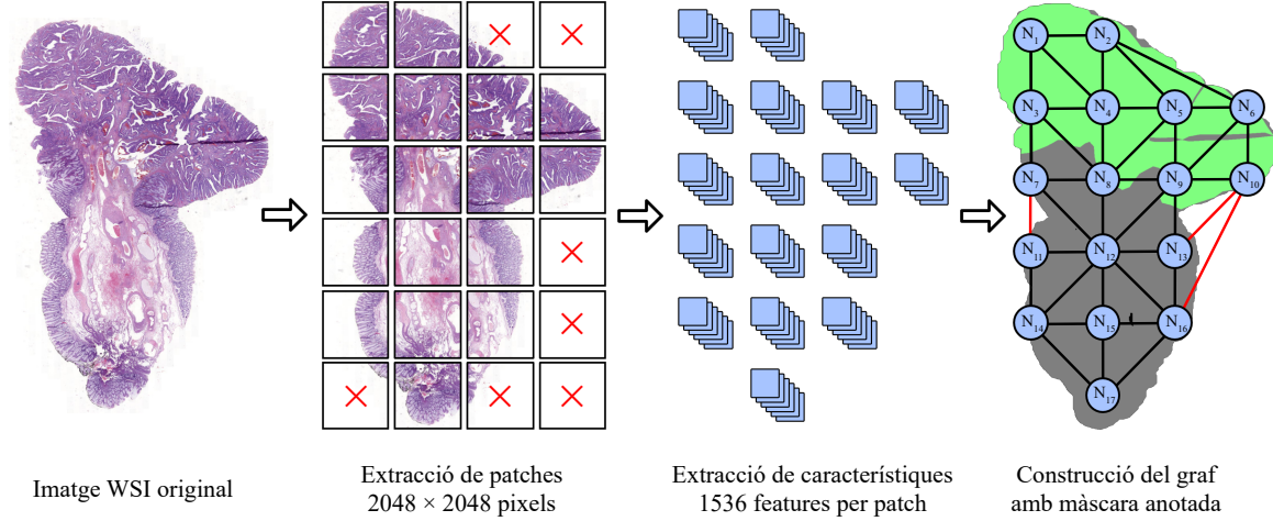
Fig. 1: Etapes del preprocessament per a la construcció del graf. D'esquerra a dreta: WSI original → extracció de patches de 2048×2048 px per finestra lliscant + filtratge → extracció de l'embedding CLS de forma [1, 1536] per UNI2 (un vector per patch ) → construcció del graf de Delaunay sobre la màscara anotada, on les arestes en vermell han estat eliminades pel filtre de màscara
