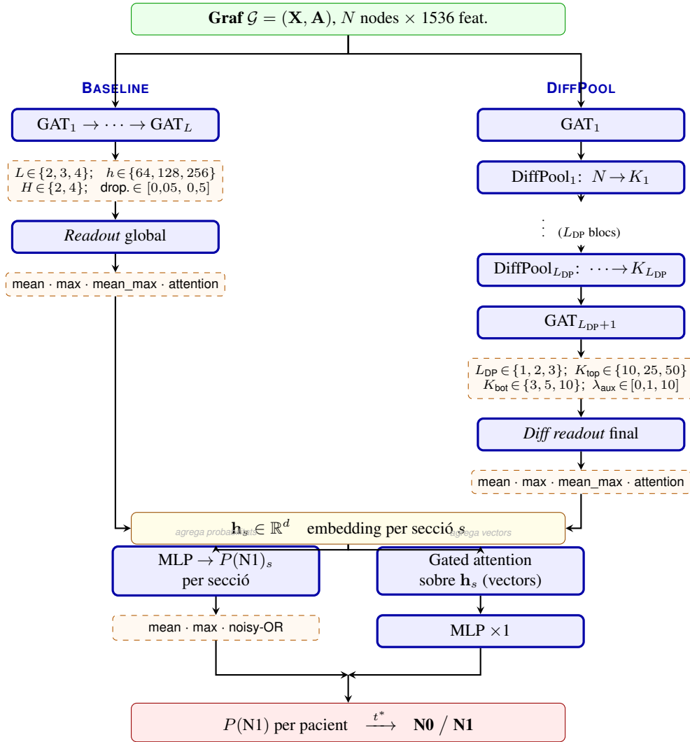
Fig. 6: Variants d'arquitectura del GATClassifier : el mateix graf \mathcal{G} es pot processar per dues branques configurables (BASELINE o DIFFPOOL), cadascuna amb la seva pròpia estratègia de readout intra-secció (caixes taronges discontinües). Totes dues convergeixen en un embedding \mathbf{h}_s per secció. L'agregació MIL bifurca de nou: mean/max/noisy-OR apliquen el MLP per secció per obtenir P(\mathbf{N1})_s i n'agreguen els escalars ; attention (gated) agrega primer els vectors \mathbf{h}_s (amb pesos d'atenció apresos) i aplica el MLP una sola vegada . L : capes GAT; h : dim. oculta; H : caps d'atenció; L_{\text{DP}} : blocs DiffPool; K_\ell : super-nodes per nivell; \lambda_{\text{aux}} : pes de la pèrdua auxiliar de DiffPool; t^* : llindar derivat del val set (Secció 7.3).
