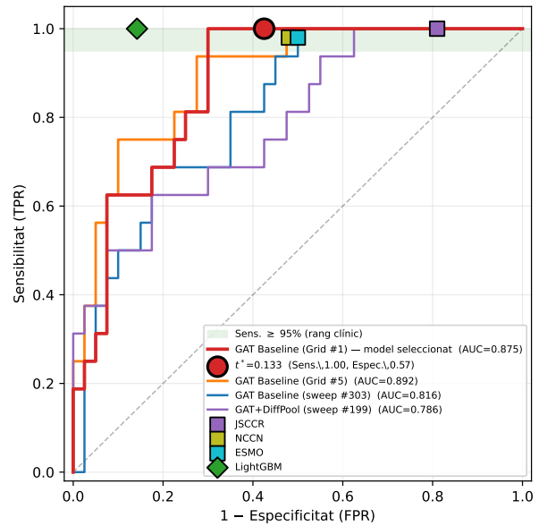
Fig. 4: Corbes ROC al conjunt de test (56 pacients) dels models comparats: Grid #1 (GAT Baseline; model seleccionat; AUC = 0,875), Grid #5 (AUC = 0,892), sweep Baseline #303 (AUC = 0,816) i sweep DiffPool #199 (AUC = 0,786). El cercle gros marca el llindar t^* = 0,133 del model seleccionat (Grid #1), que assoleix \text{sens.} = 100\% i \text{espec.} = 57,5\% al test. t^* s'ha derivat exclusivament del val set sense data leakage . Es marquen els punts operatius publicats de JSCCR, NCCN, ESMO (quadrats) i LightGBM (diamant).
