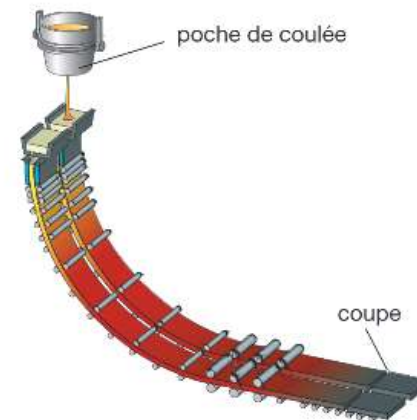
machine courbe avec cintrage
