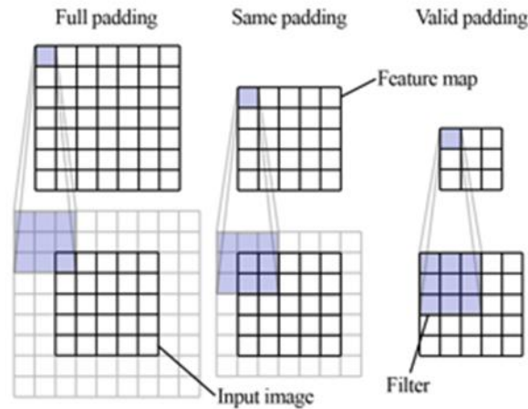
الشكل 7-2: الفرق بين أنواع الـ Padding الثلاث.
