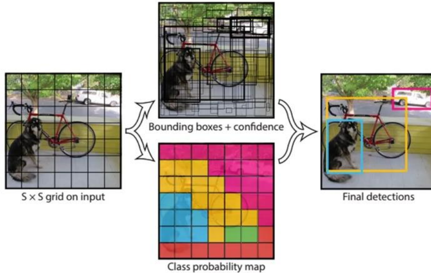
الشكل 13-2: النتيجة النهائية للكشف باستخدام YOLO.
