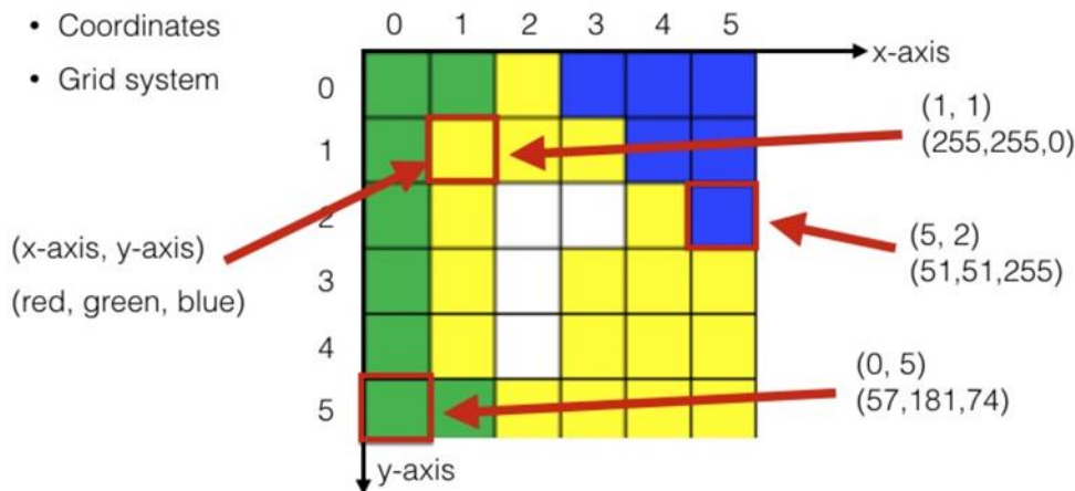
الشكل 1-2: جزء من الصورة الرقمية.
