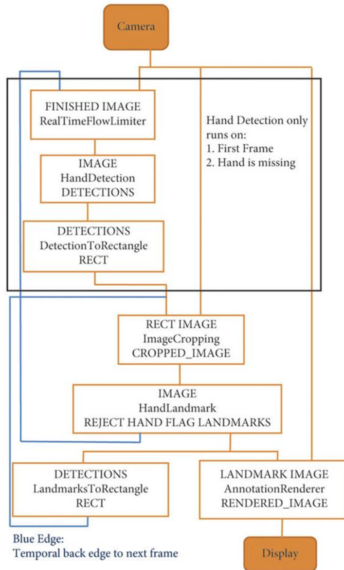
الشكل 3-5: تسلسل مراحل معالجة الصورة في نظام MediaPipe Hands.
