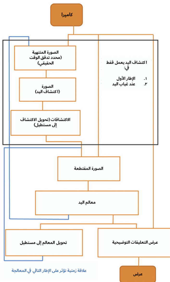
الشكل 5-3: مراحل معالجة الصورة في نظام MediaPipe Hands.
