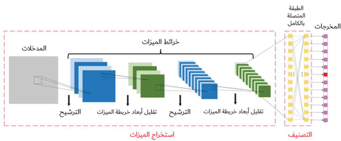
الشكل 10-2: آلية عمل شبكة CNN.
