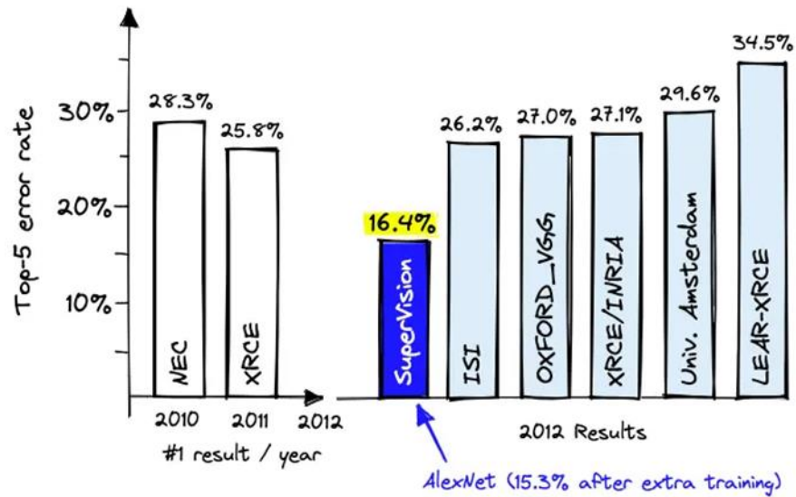
الشكل 2-7: تطور نماذج التعلم العميق.
