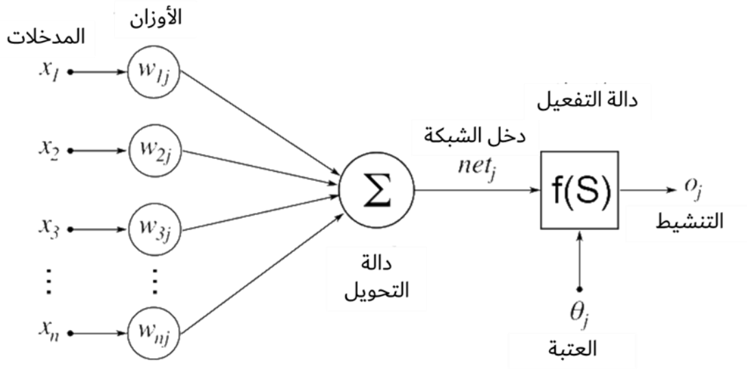
الشكل 8-2: آلية عمل الشبكة العصبية الاصطناعية.
