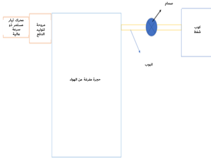
الشكل 1-3: التمثيل التخطيطي لآلية الشفط.
