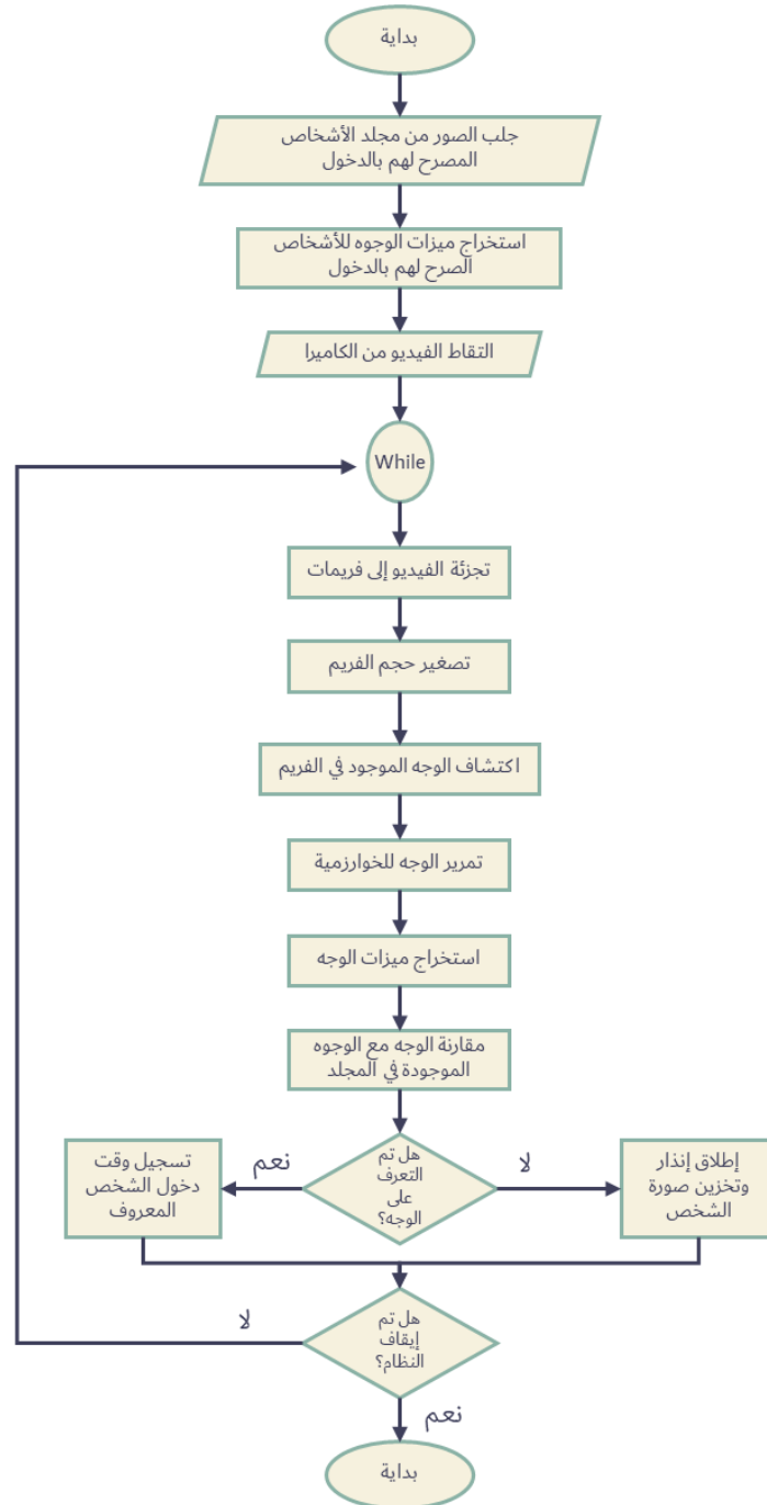
الشكل 1-4: المخطط التدفقي (الخوارزمية) الخاصة بنظام التحكم بالدخول.
