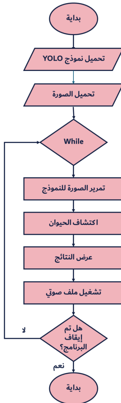
الشكل (5-1): المخطط التدفقي لوظيفة التعرف على الحيوانات.
