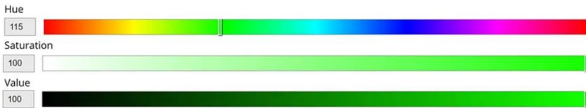
الشكل (3-4): تأثير تغيير التشبع والضوء على الألوان في نموذج HSV.
