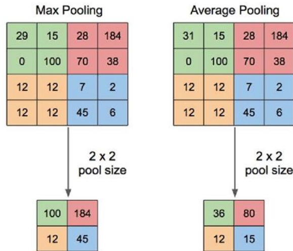
الشكل (2-8): الفرق بين Max Pooling و Average Pooling.
