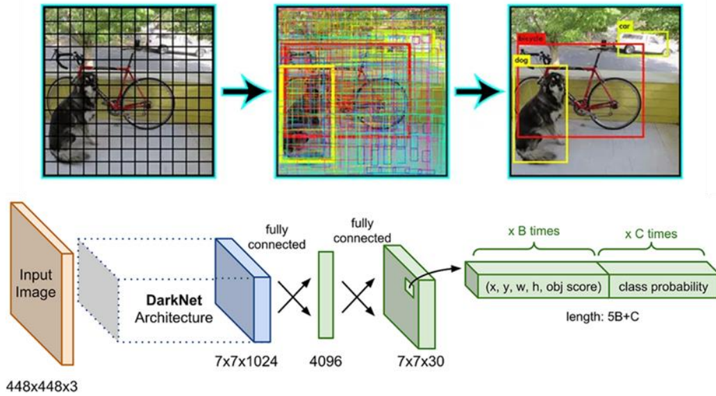
الشكل (9-3): هيكل خوارزمية YOLO.
