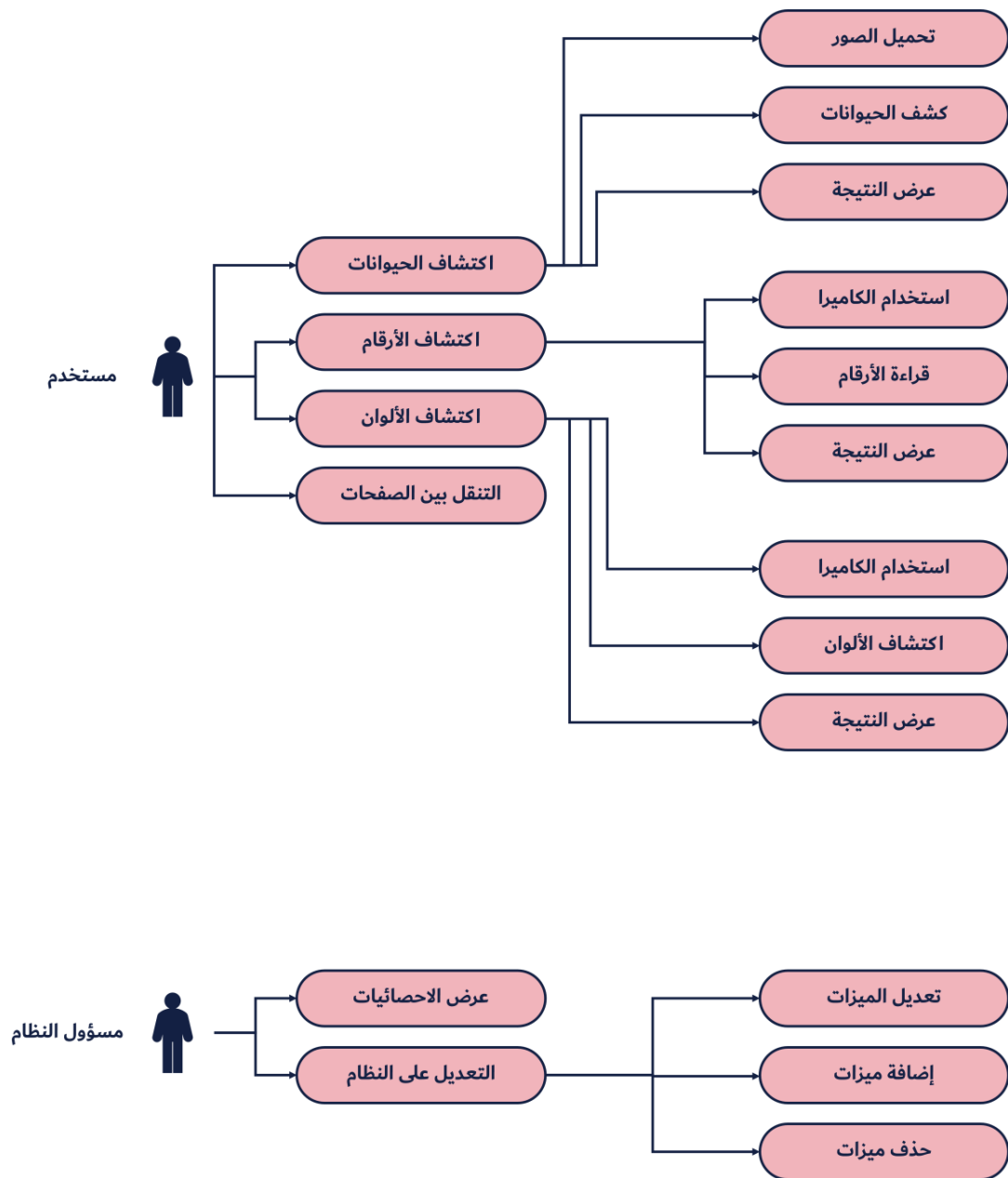
الشكل (4-7): مخطط حالات الاستخدام.
