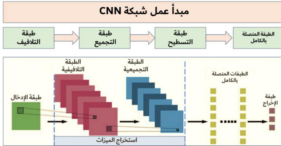
الشكل (2-6): خطوات عمل شبكة CNN.
