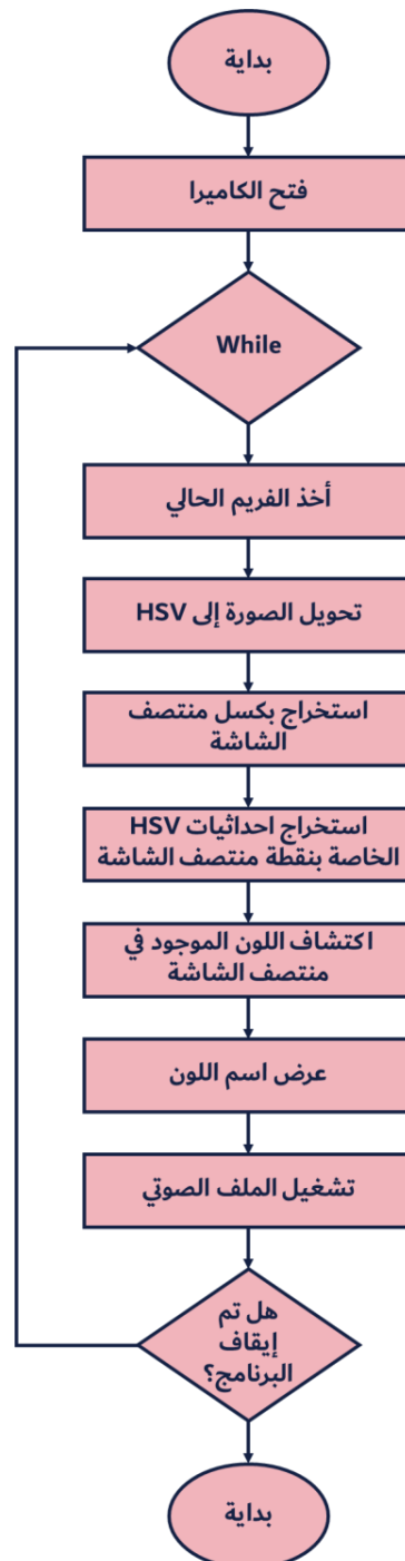
الشكل (2-5): المخطط التدفقي لوظيفة التعرف على الألوان.
