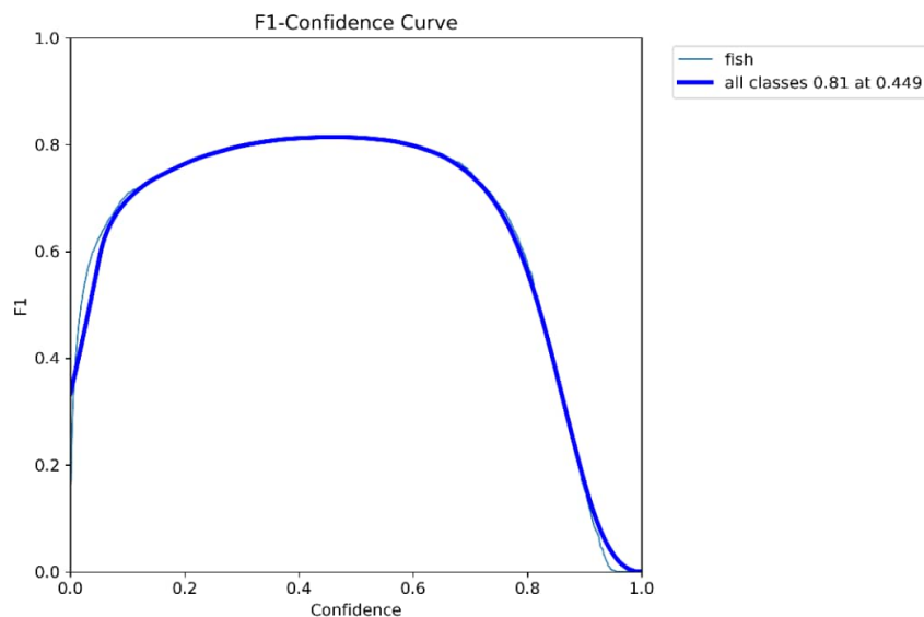
الشكل (5-29): منحنى F1 - الثقة لنموذج كشف الأسماك.
