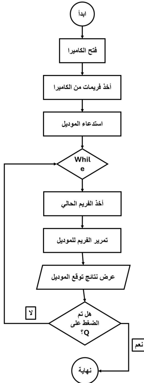
[الشكل 4-1]: مخطط خوارزمية العمل.
