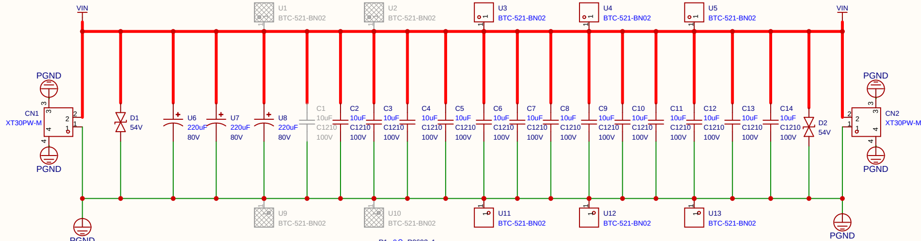
电源输入滤波
