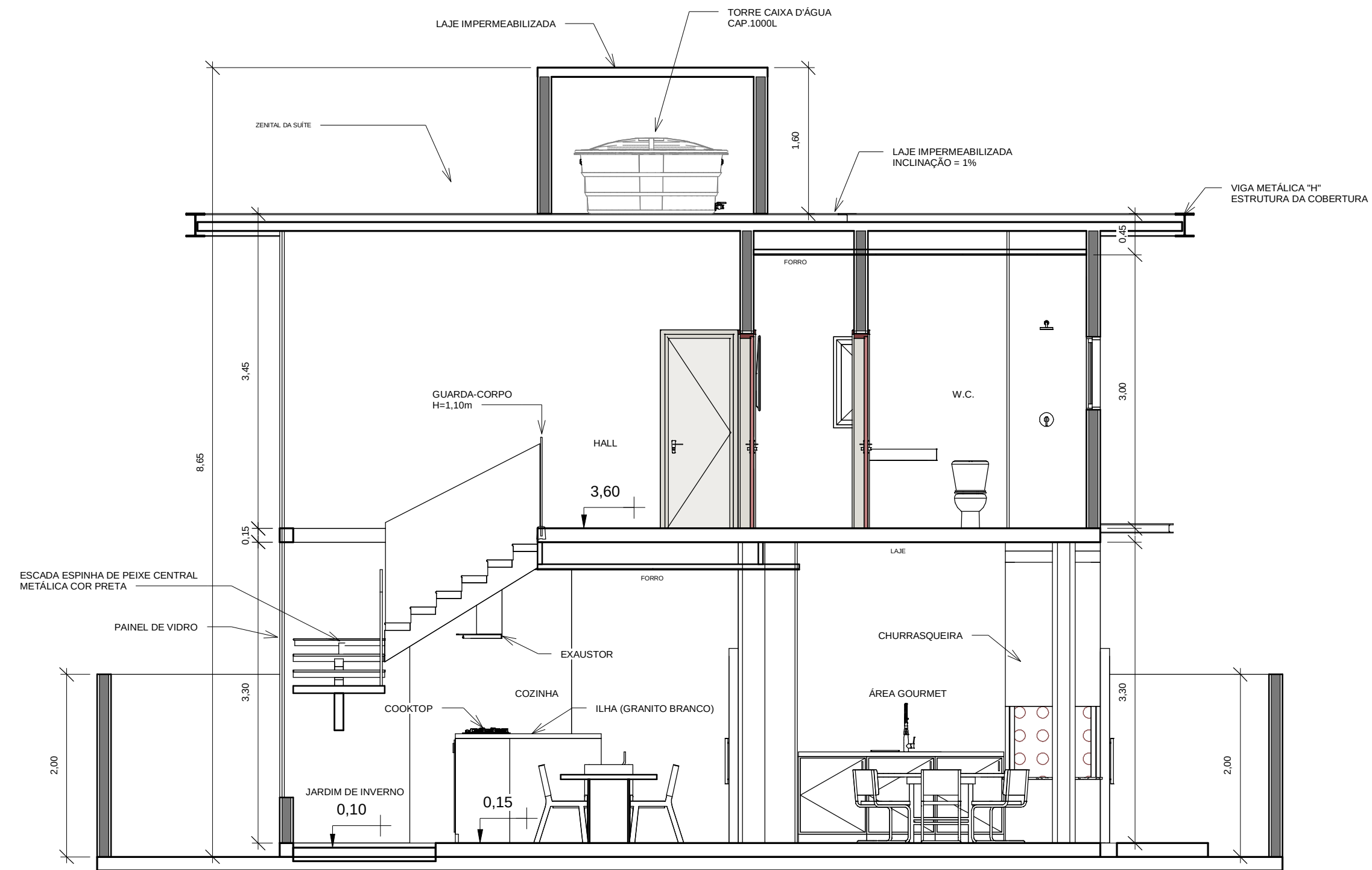
2 CORTE BB 1 : 50
