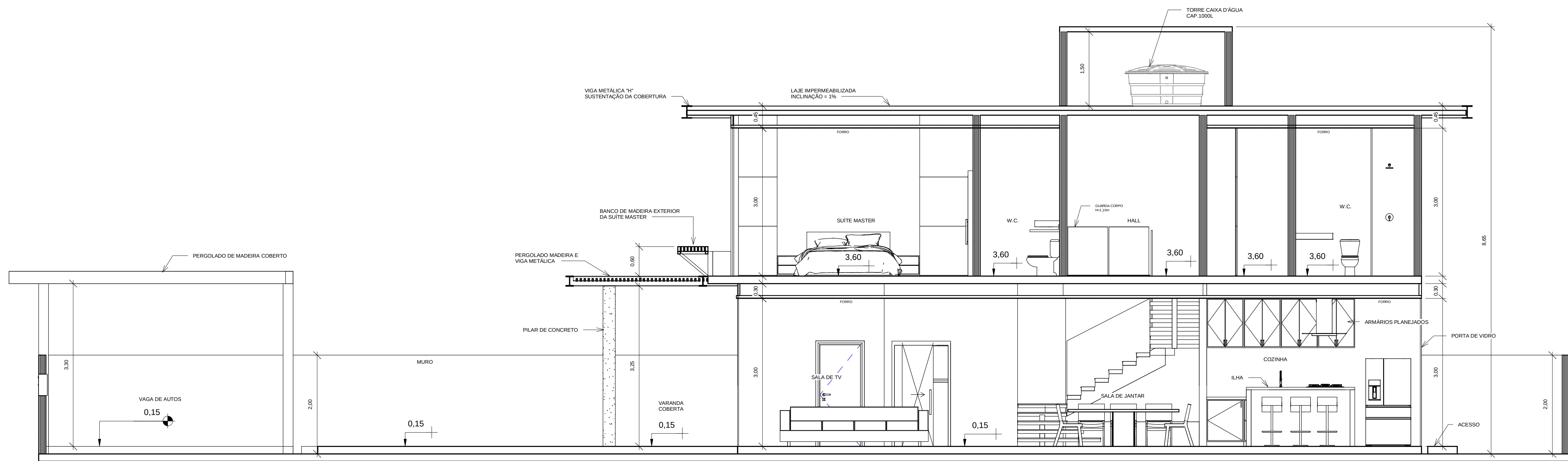
1 CORTE AA 1 : 50
