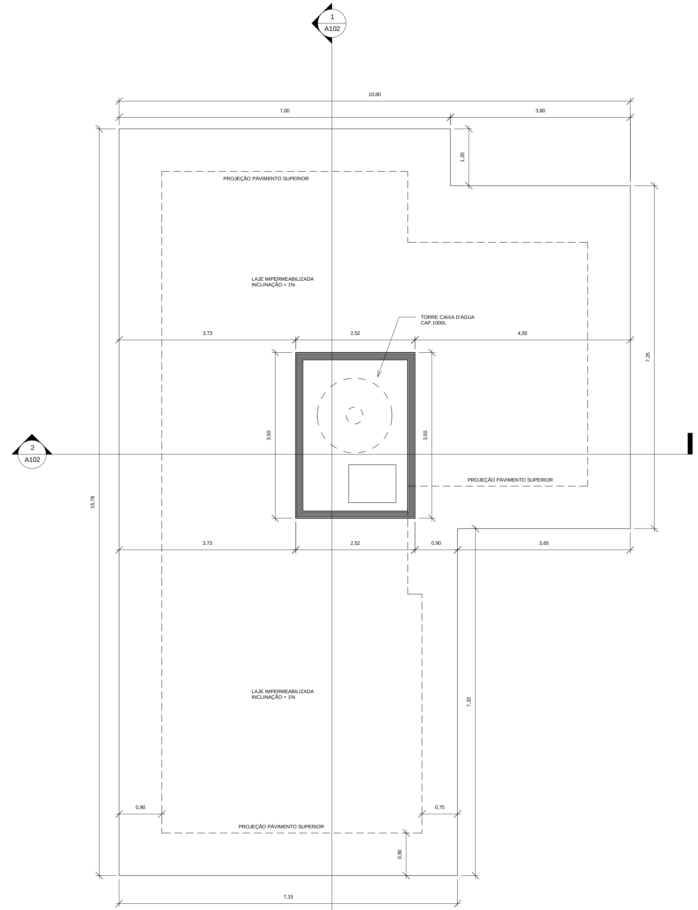
3 COBERTURA 1 : 50
