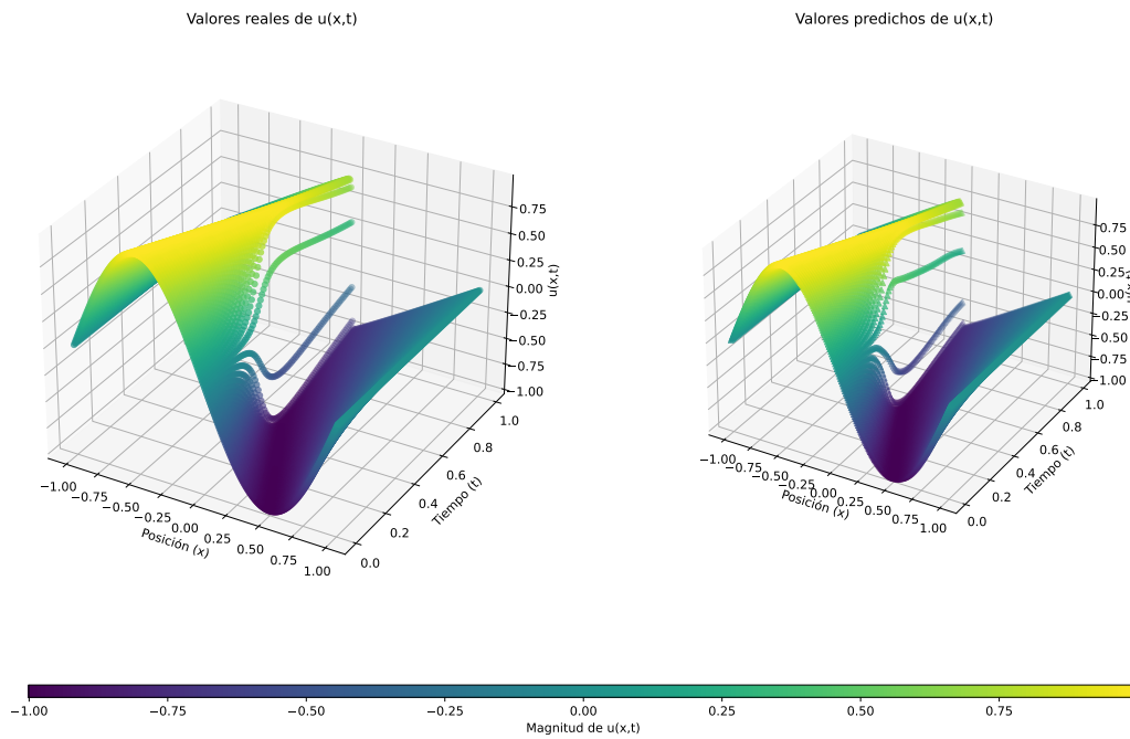
Figura 7.2.: Comparación entre solución real y predicción de la red neuronal para la ecuación de Burger 1D. Debido a su naturaleza unidimensional, es posible plasmar en un eje al tiempo ( t ) y representar a la función a lo largo de éste como una serie de fotos para un instante t dado.
