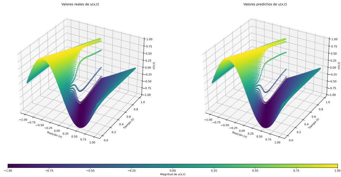
Figura 7.2.: Comparación entre solución real y predicción de la red neuronal para la ecuación de Burger 1D. Debido a su naturaleza unidimensional, es posible plasmar en un eje al tiempo ( t ) y representar a la función a lo largo de éste como una serie de fotos para un instante t dado.
