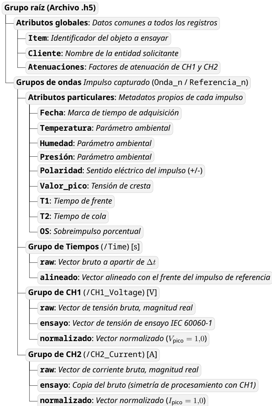
Figura 5.2: Estructura jerárquica de la base de datos.
