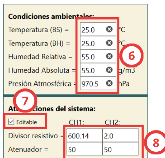
Figura 6.13: Edición de campos a completar.
