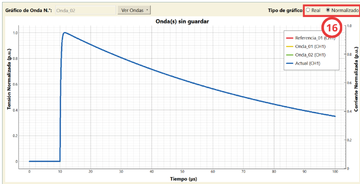
Figura 6.19: Gráfico normalizado a valor unitario.
