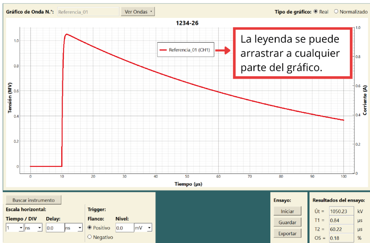
Figura 6.17: Ejemplo de onda guardada.
