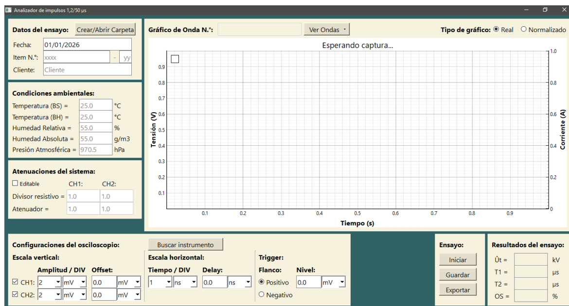
Figura 6.1: GUI en tamaño 1366x768 px.
