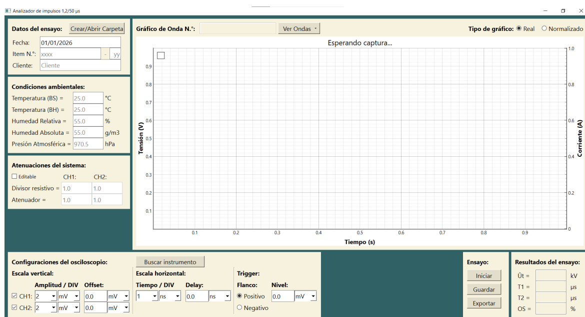
Figura 6.2: GUI en tamaño 1920x1080 px.
