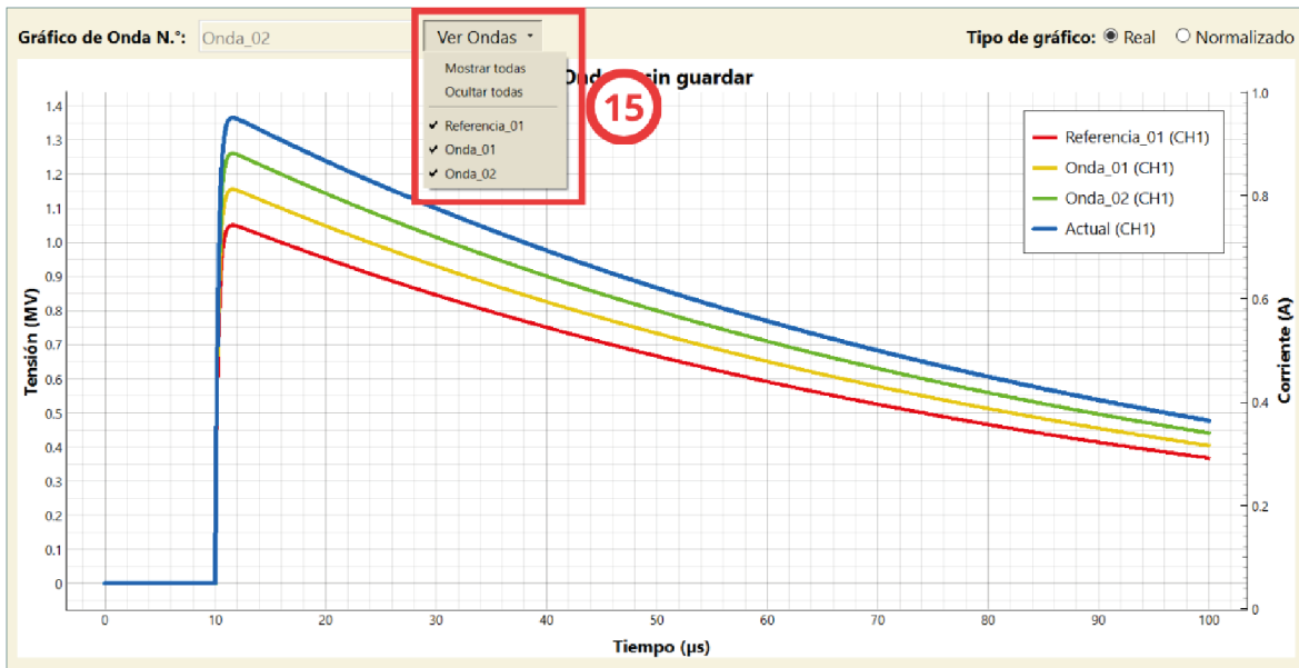
Figura 6.18: Historial de impulsos guardados.
