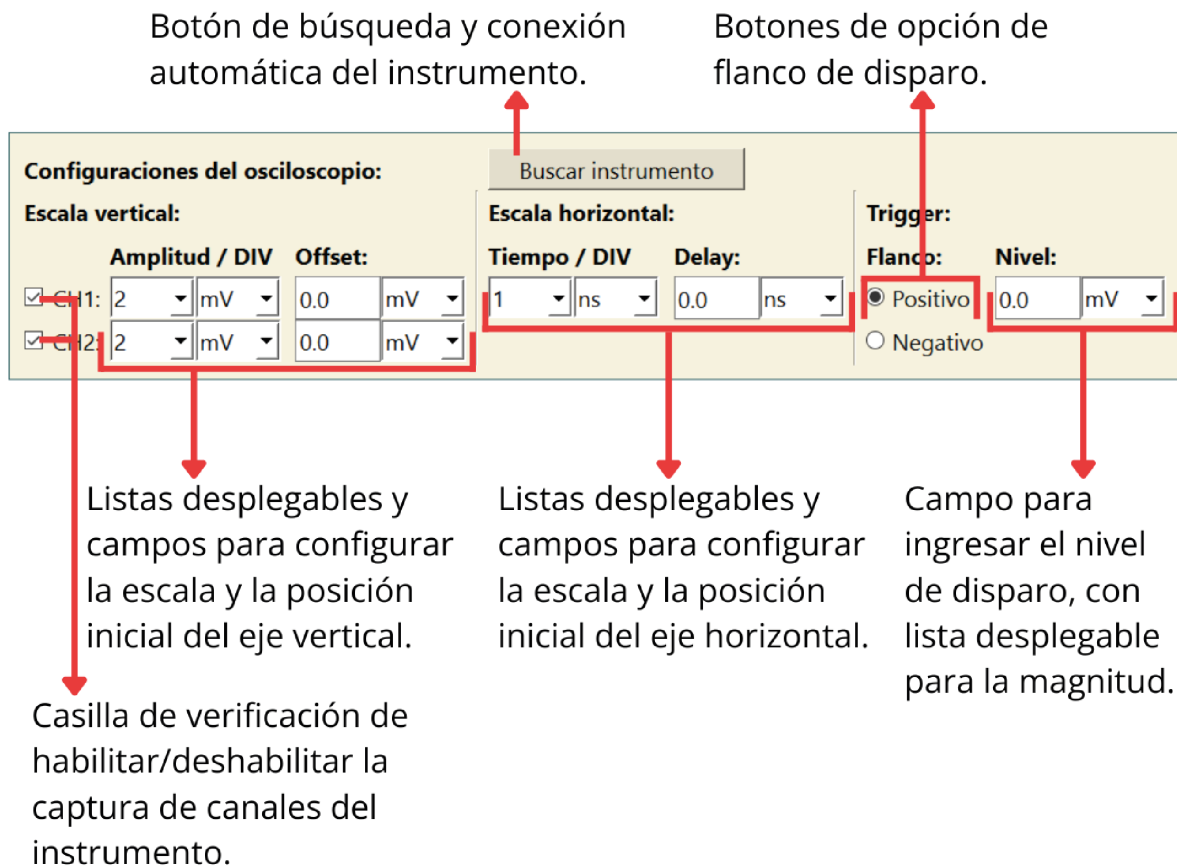
Figura 6.7: Bloque de Control del instrumento.
