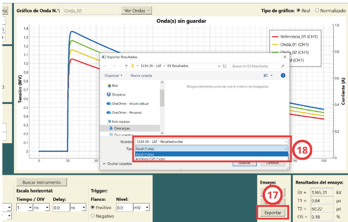
Figura 6.20: Ejemplo de exportación de resultados.
