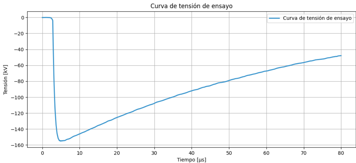
Figura 8.9: Curva de tensión de ensayo U_t[n] . Fuente: Propia.
