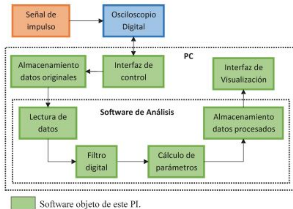
Figura 4 – Diagrama de bloques del software. Fuente: Propia
