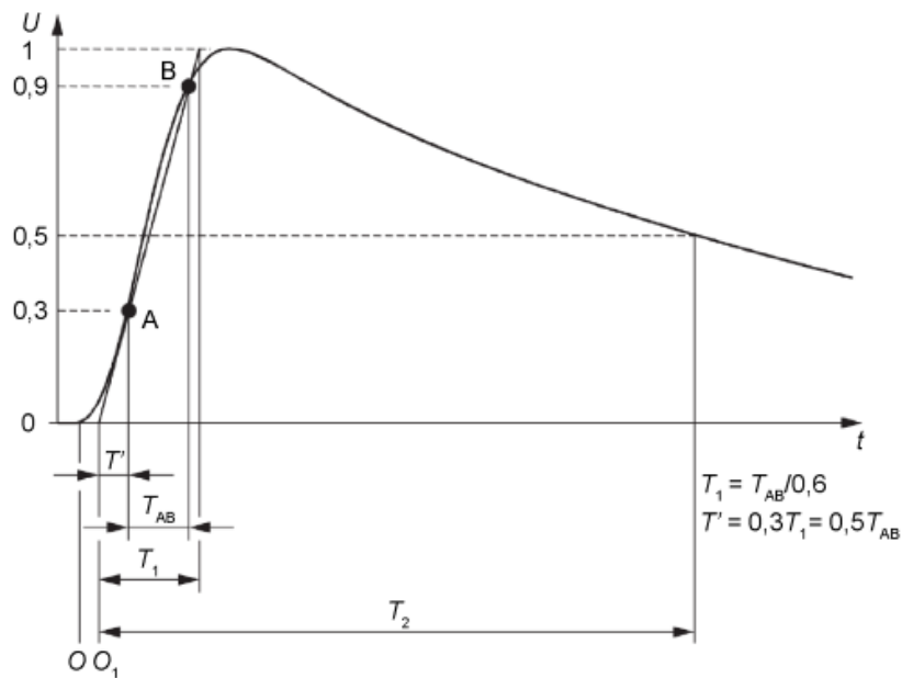
Figura 2.6: Parámetros de tiempo del impulso de tensión tipo rayo pleno. Fuente: [4].
