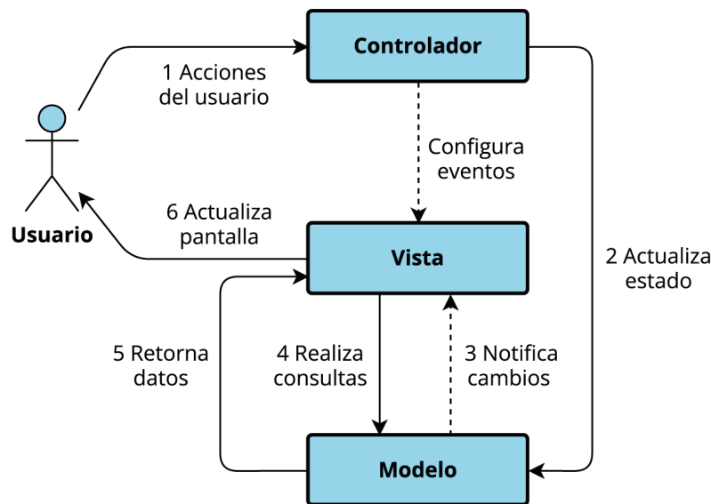
Figura 5.1: Interacciones entre módulos del esquema MVC. Fuente: Propia.
