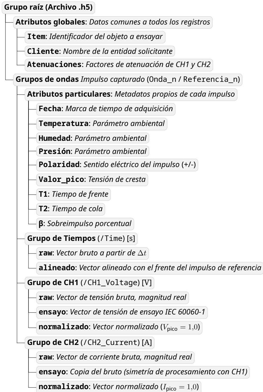
Figura 7.11: Estructura jerárquica de la base de datos. Fuente: Propia.
