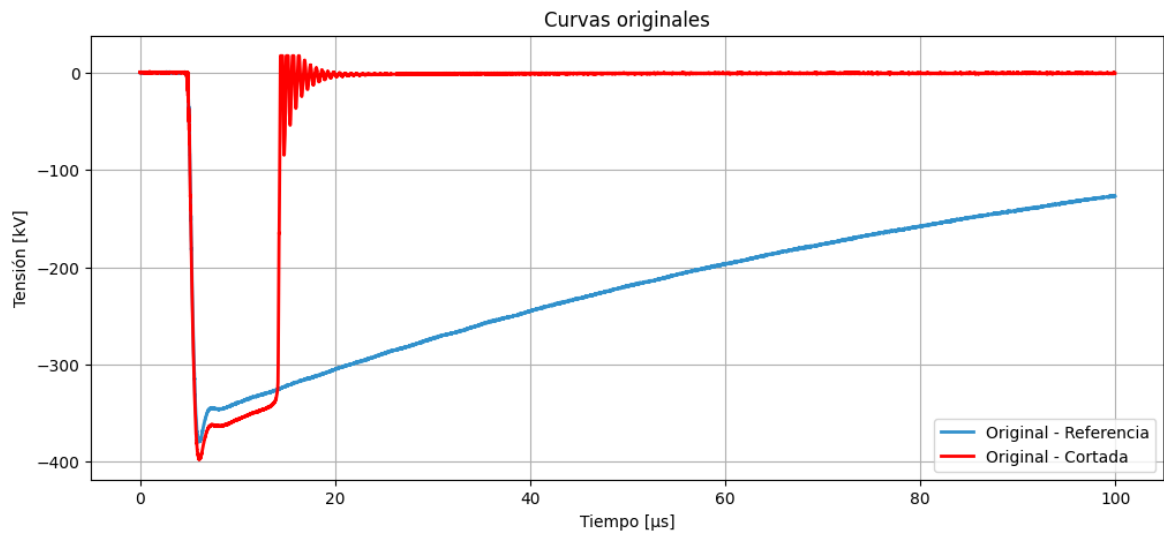
Figura 8.11: Señales originales del TDG (Referencia plena y onda cortada). Fuente: Propia.
