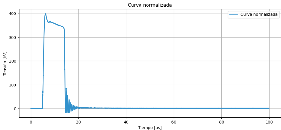
Figura 8.13: Normalización de polaridad. Fuente: Propia.
