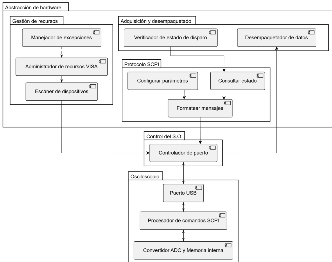
Figura 7.4: Diagrama de componentes de la HAL. Fuente: Propia.
