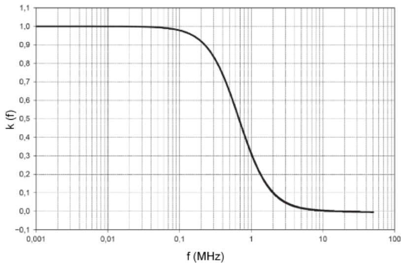
Figura 2.3: Función tensión de ensayo. Fuente: [4].
