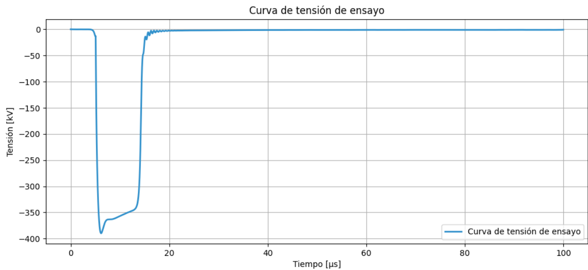
Figura 8.18: Curva de tensión de ensayo U_t[n] . Fuente: Propia.
