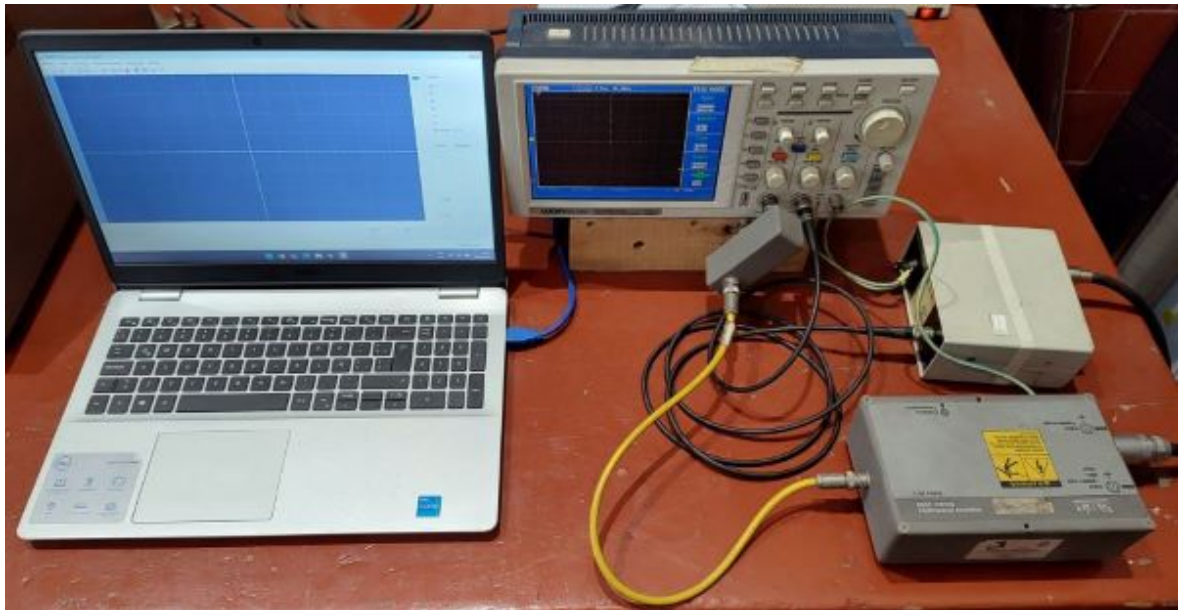
Figura 2.10: Sistema de adquisición compuesto por notebook, osciloscopio y dos atenuadores coaxiales. Fuente: Propia.
