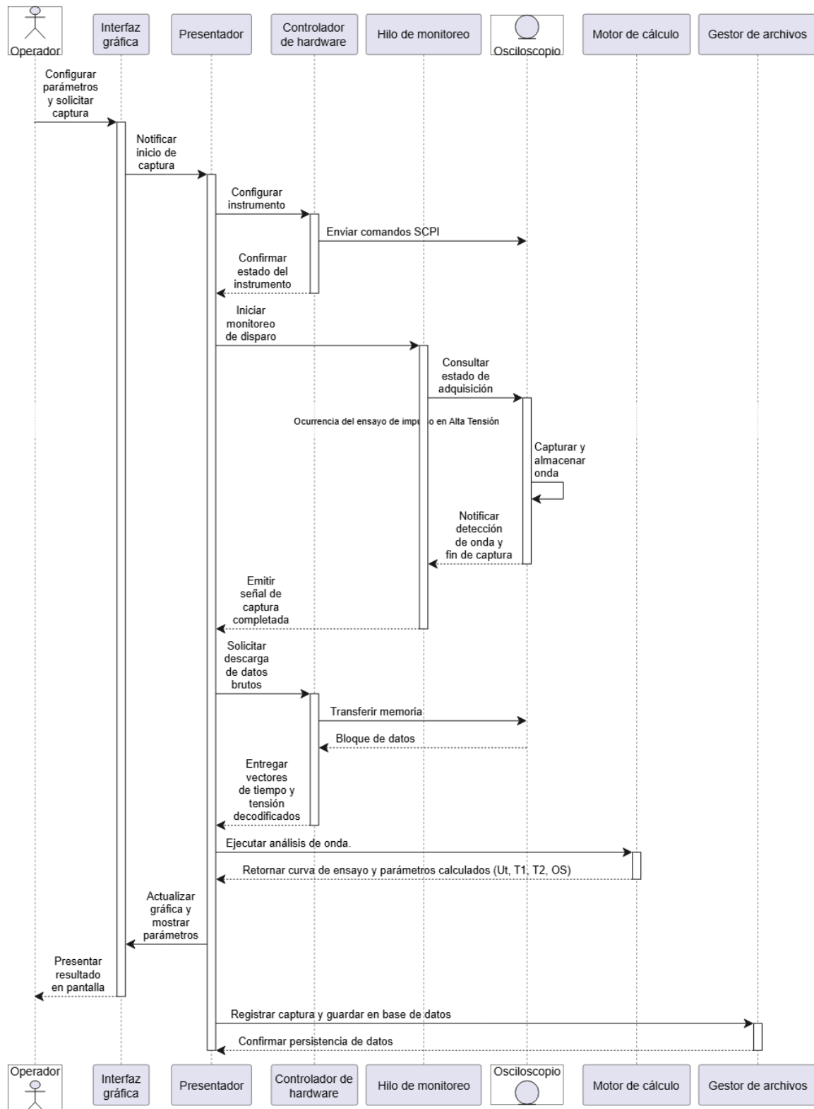
Figura 7.5: Diagrama de secuencia de la captura de impulsos. Fuente: Propia.
