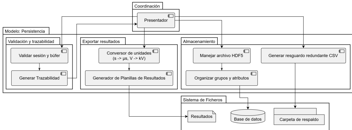
Figura 7.7: Diagrama de componentes del gestor de la base de datos. Fuente: Propia.
