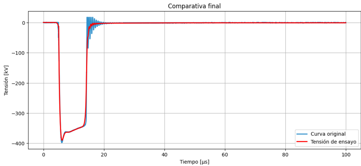
Figura 8.19: Comparativa entre la curva de tensión de ensayo procesada y la original bruta. Fuente: Propia.
