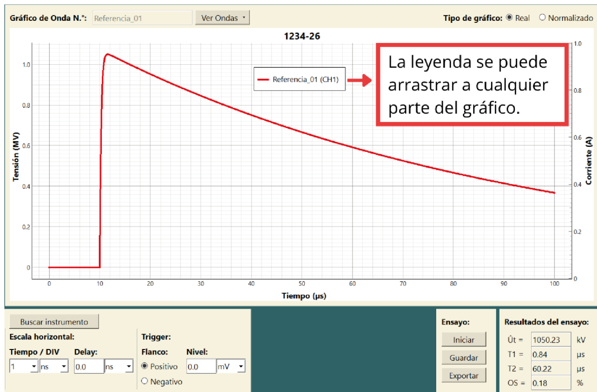
Figura 7.28: Ejemplo de onda guardada. Fuente: Propia.
