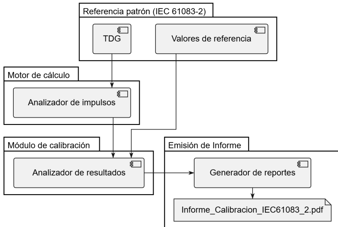
Figura 8.1: Diagrama de componentes del sistema de calibración. Fuente: Propia.
