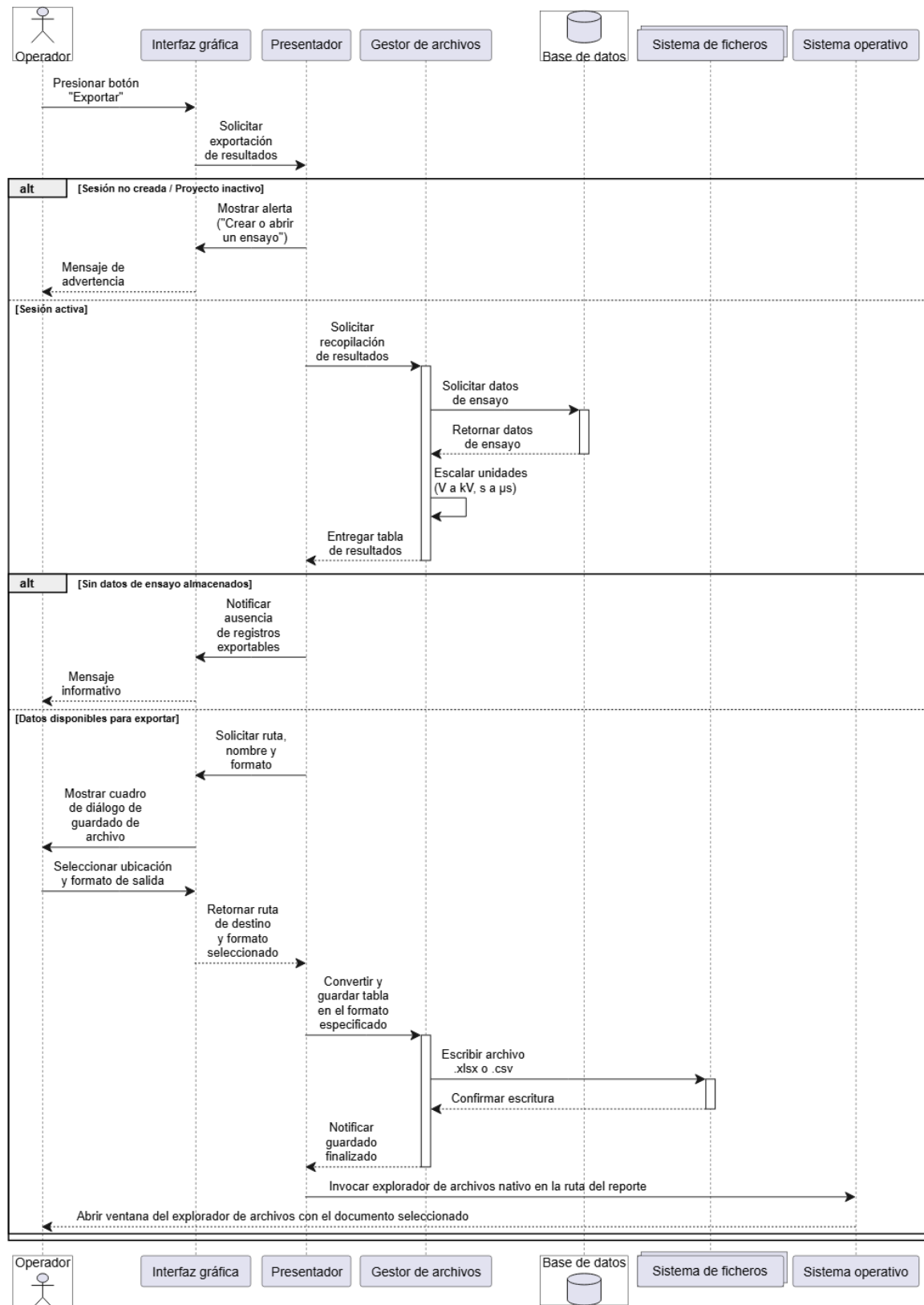
Figura 7.9: Diagrama de secuencia de la exportación de impulsos. Fuente: Propia.
