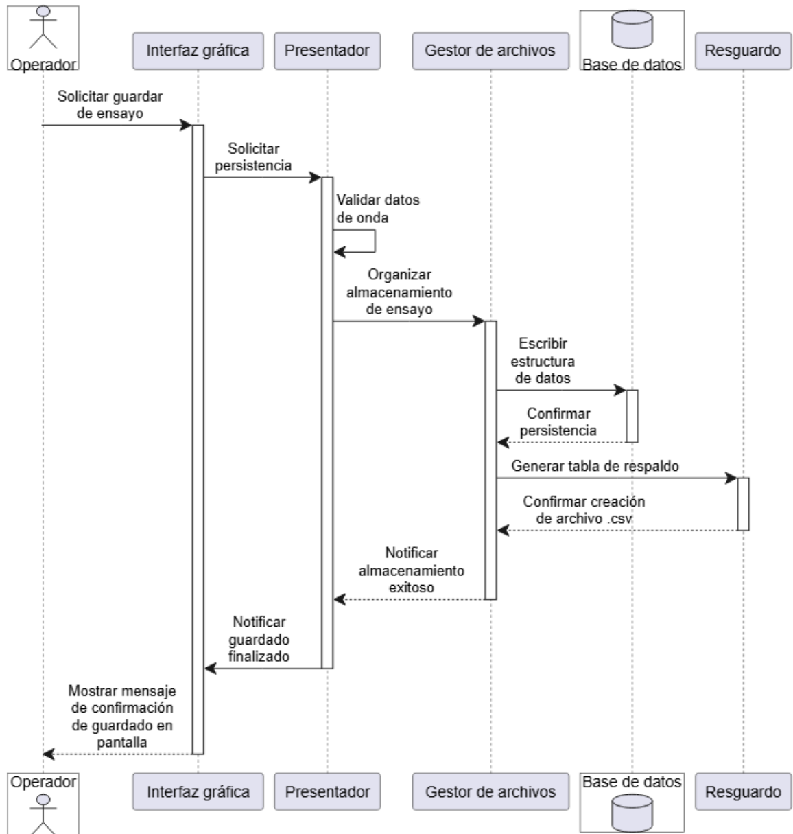
Figura 7.8: Diagrama de secuencia del guardado de información. Fuente: Propia.
