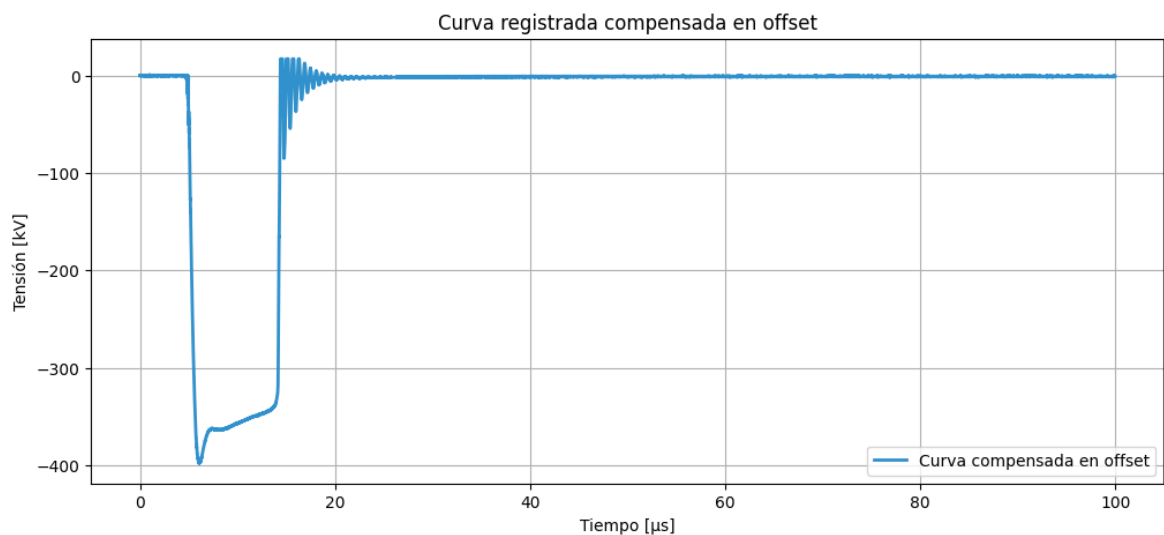
Figura 8.12: Acondicionamiento de continua de la onda cortada. Fuente: Propia.
