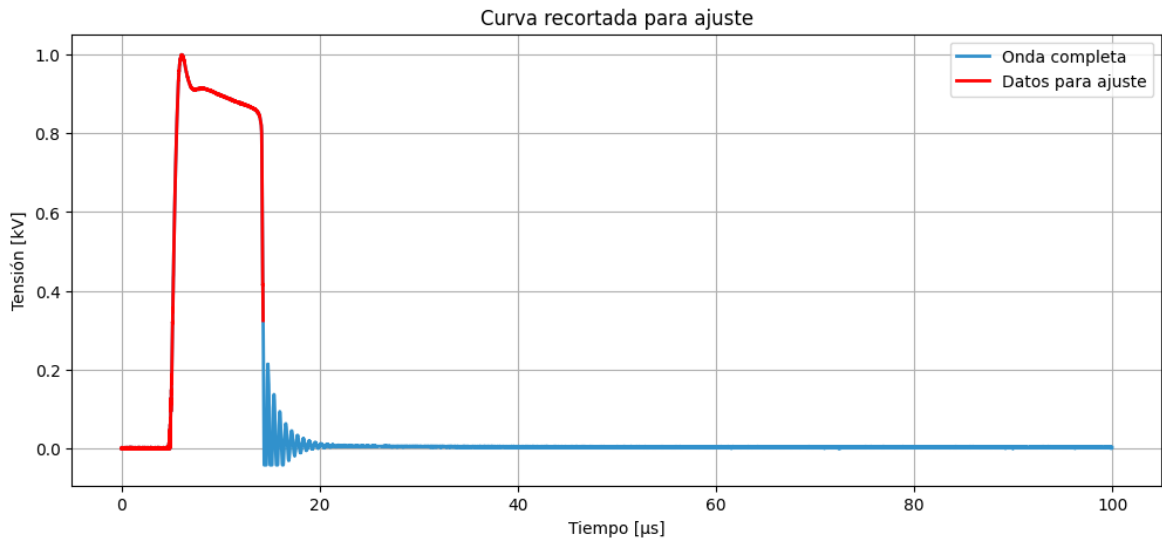
Figura 8.14: Segmentación del frente para el cálculo del factor de escala. Fuente: Propia.
