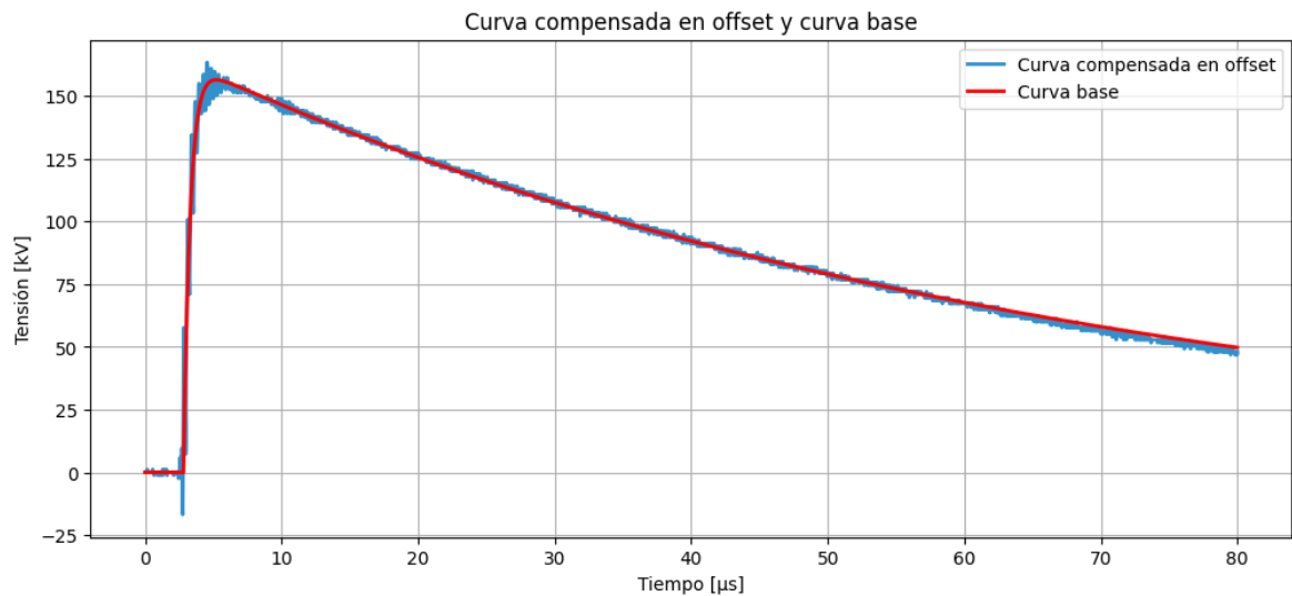
Figura 8.6: Sintetización de la curva base. Fuente: Propia.
