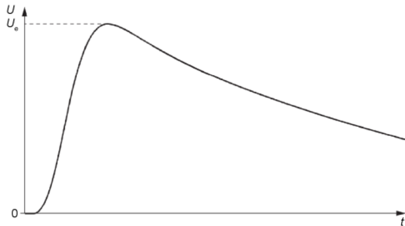
Figura 2.1: Impulso de tensión tipo rayo pleno. Fuente: [4].
