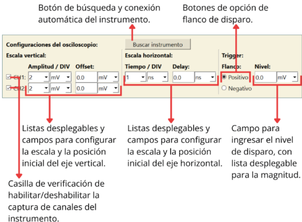
Figura 7.18: Bloque de Control del instrumento. Fuente: Propia.
