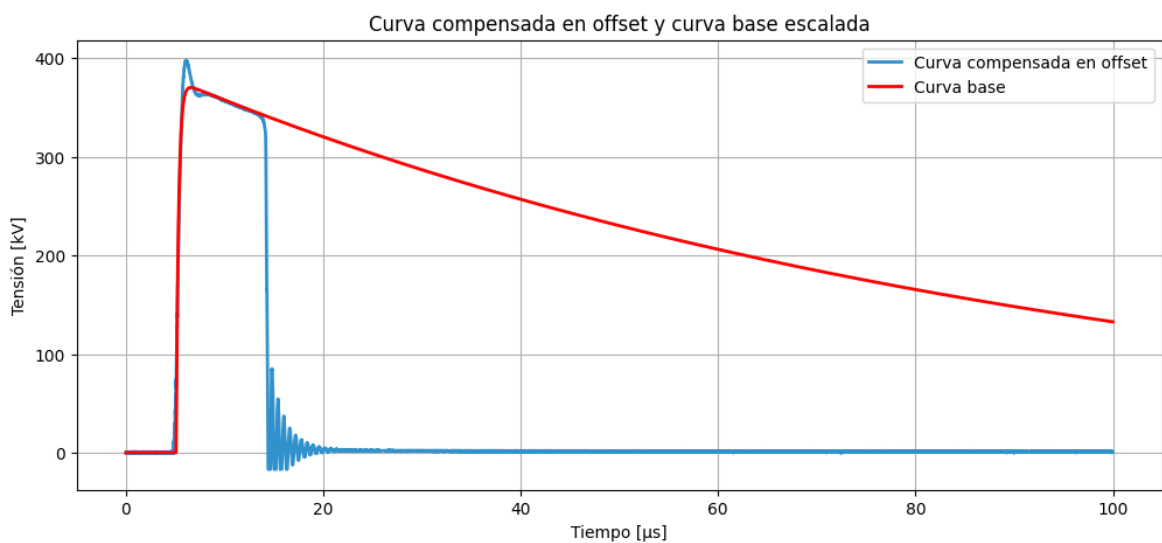
Figura 8.15: Sintetización de la curva base escalada analíticamente. Fuente: Propia.
