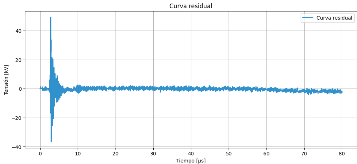
Figura 8.7: Curva residual obtenida. Fuente: Propia.
