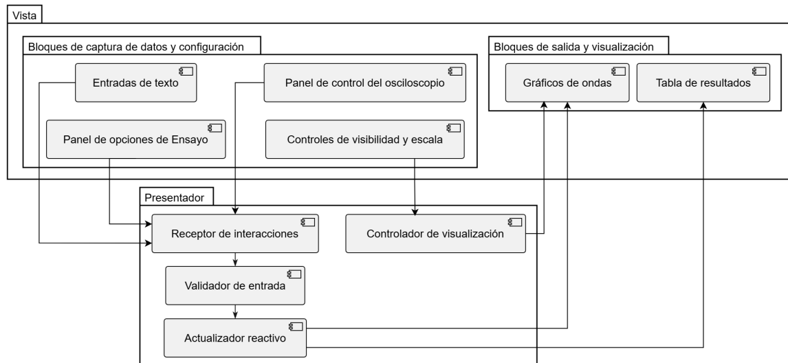
Figura 7.1: Diagrama de coordinación de la gui. Fuente: Propia.
