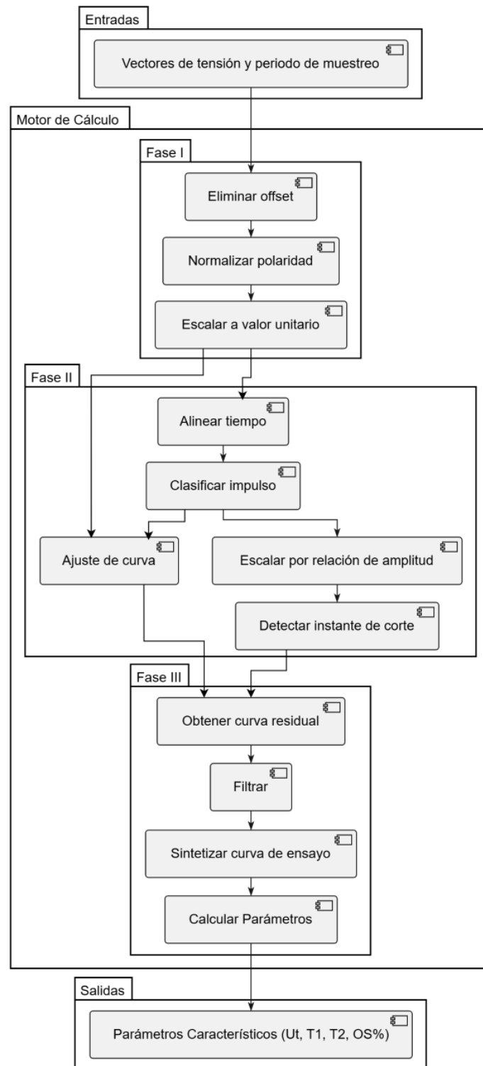
Figura 7.6: Diagrama de flujo de motor de cálculo. Fuente: Propia.
