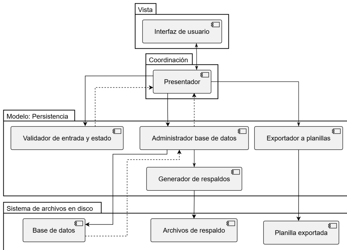
Figura 7.3: Diagrama de coordinación del gestor de archivos. Fuente: Propia.
