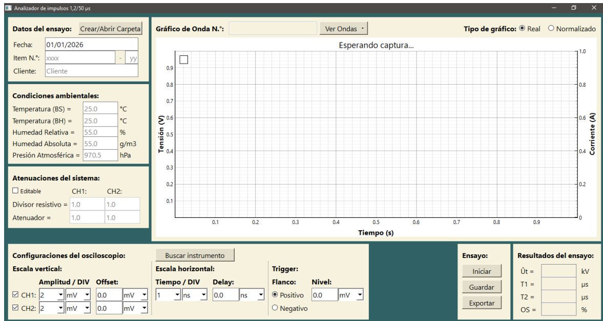
Figura 7.12: GUI en tamaño 1366x768 px. Fuente: Propia.
