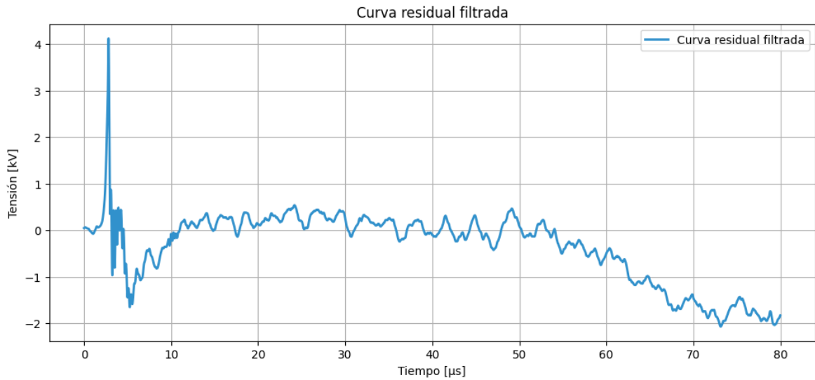
Figura 8.8: Curva residual filtrada. Fuente: Propia.
