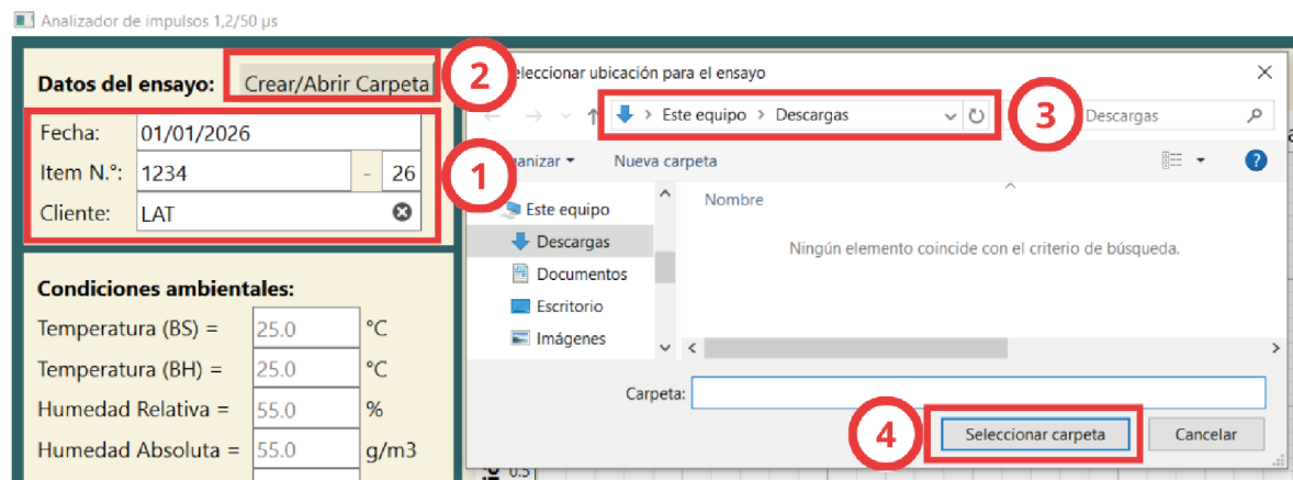
Figura 7.22: Creación de directorio del ensayo. Fuente: Propia.
