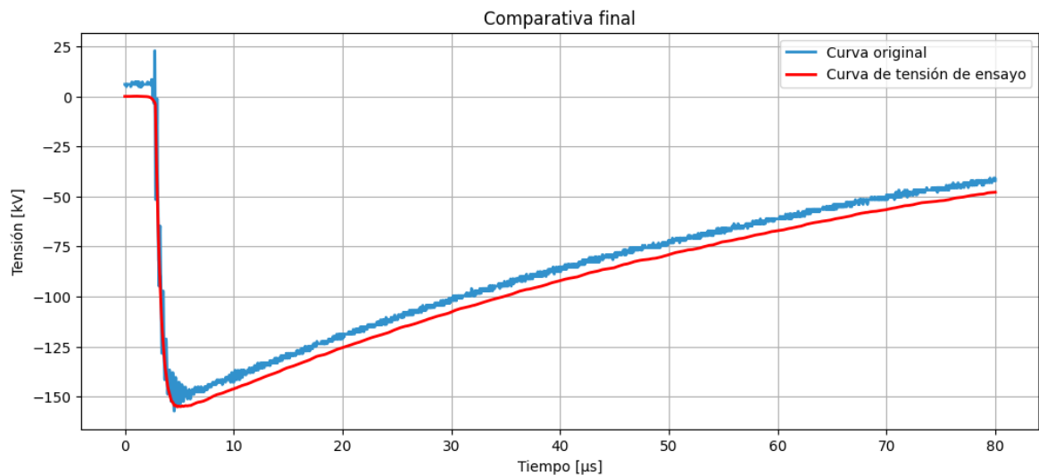
Figura 8.10: Comparativa entre la curva de tensión de ensayo y la original bruta. Fuente: Propia.
