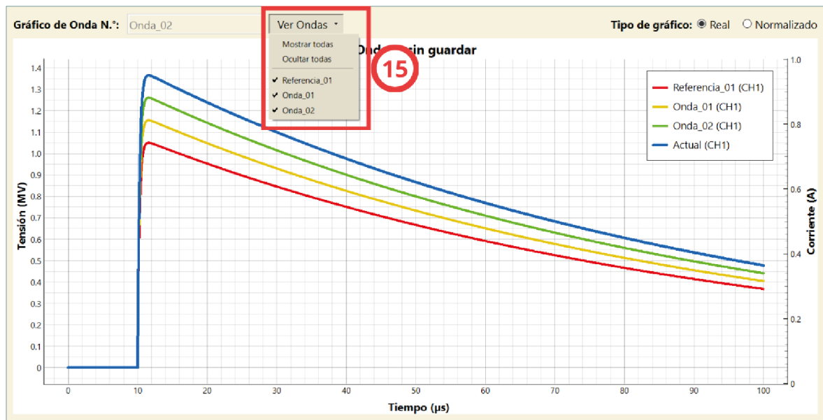
Figura 7.29: Historial de impulsos guardados. Fuente: Propia.
