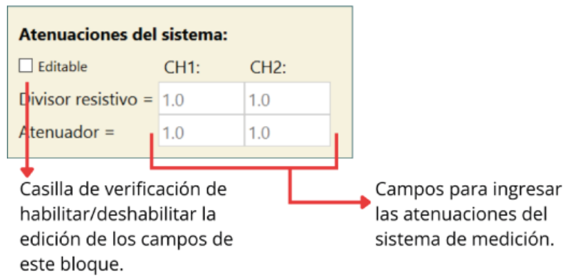
Figura 7.17: Bloque de Atenuaciones del sistema de medición. Fuente: Propia.
