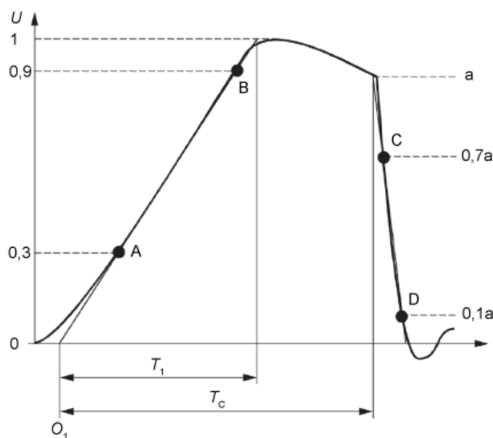
Figura 2.7: Impulso de tensión tipo rayo cortado en la cola. Fuente: [4].
