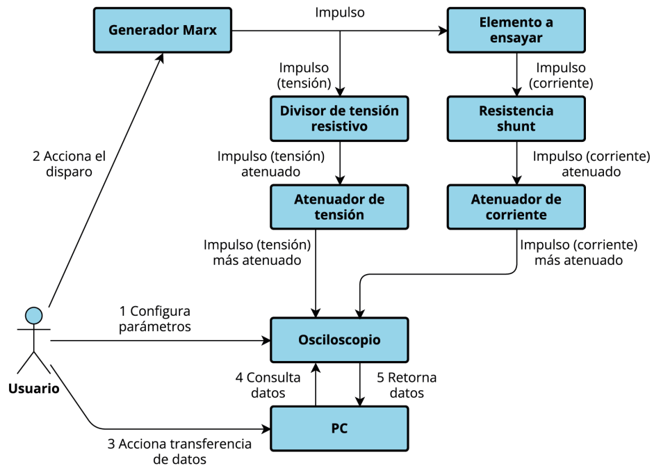
Figura 1.1: Diagrama de ensayo de impulso. Fuente: Propia.
