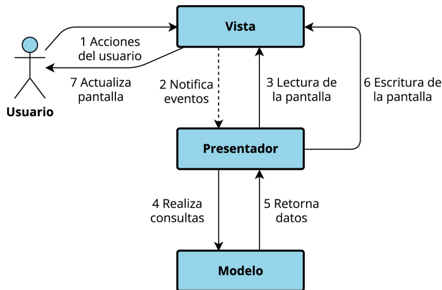
Figura 5.2: Interacciones entre módulos del esquema MVP. Fuente: Propia.
