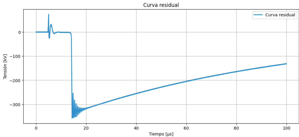
Figura 8.16: Curva residual obtenida para el impulso cortado. Fuente: Propia.
