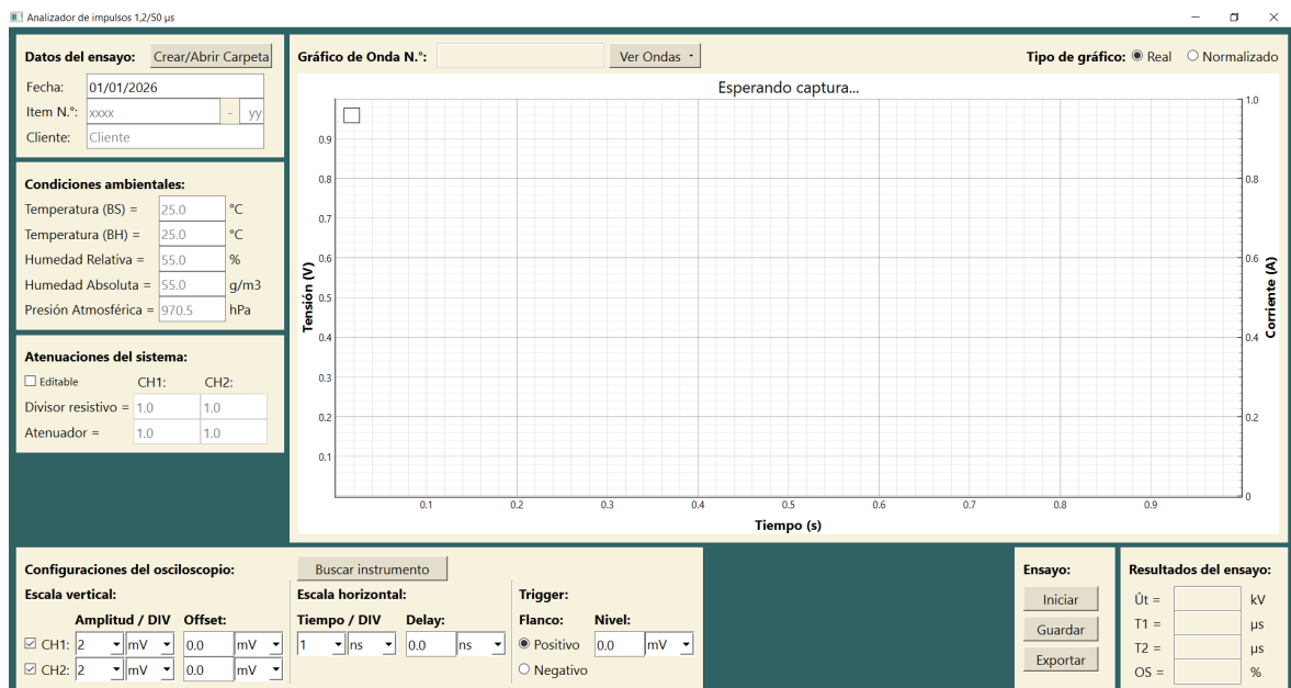
Figura 7.13: GUI en tamaño 1920x1080 px. Fuente: Propia.
