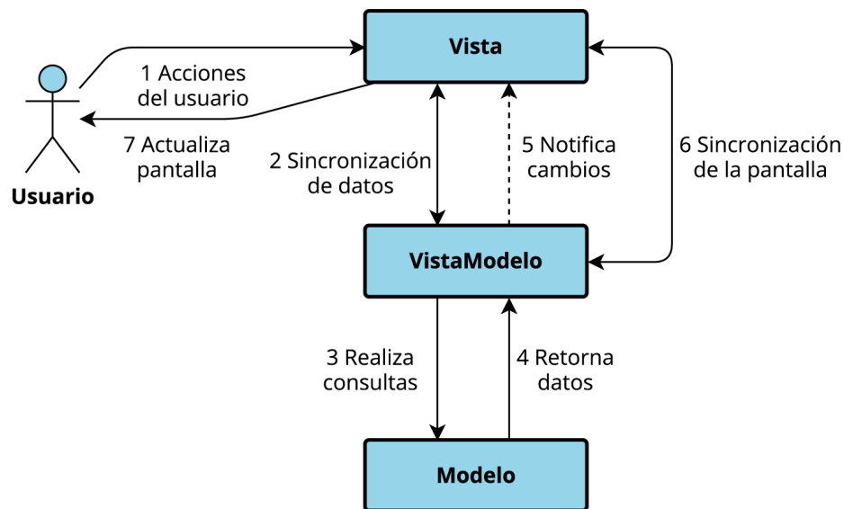
Figura 5.3: Interacciones entre módulos del esquema MVVM. Fuente: Propia.
