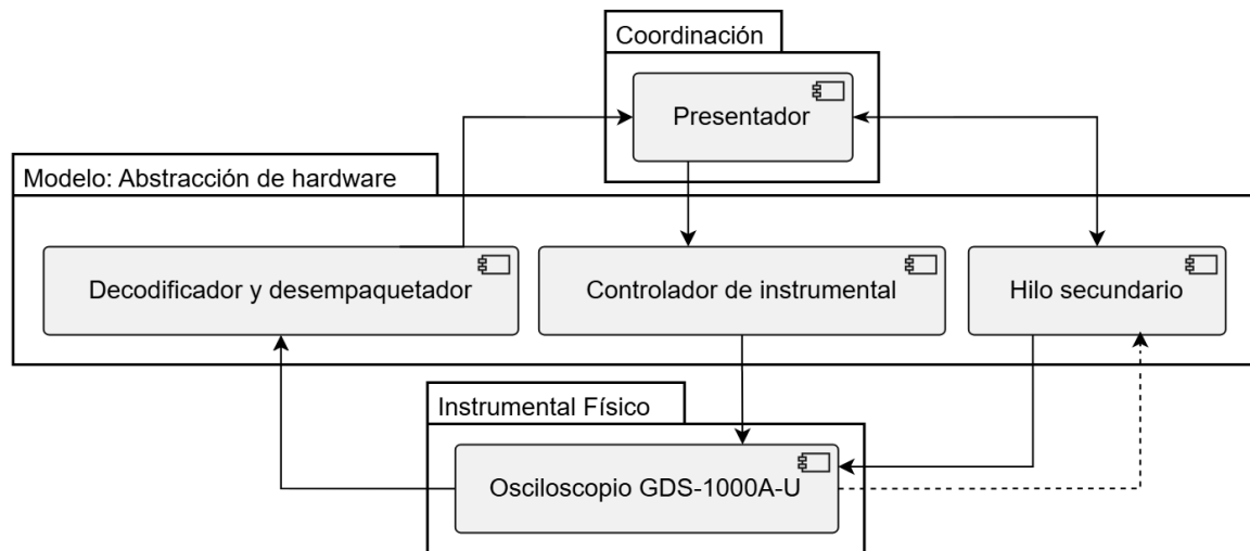
Figura 7.2: Diagrama de coordinación de la HAL. Fuente: Propia.
