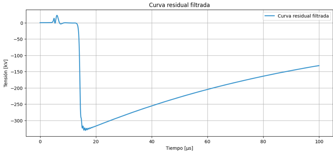
Figura 8.17: Curva residual filtrada. Fuente: Propia.
