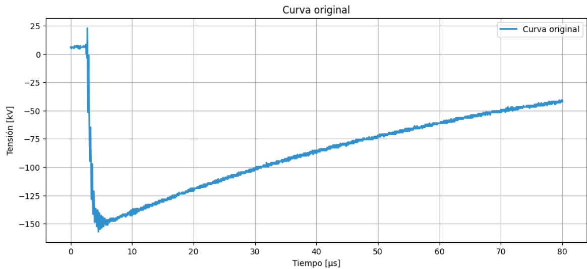
Figura 8.2: Adquisición de datos. Fuente: Propia.
