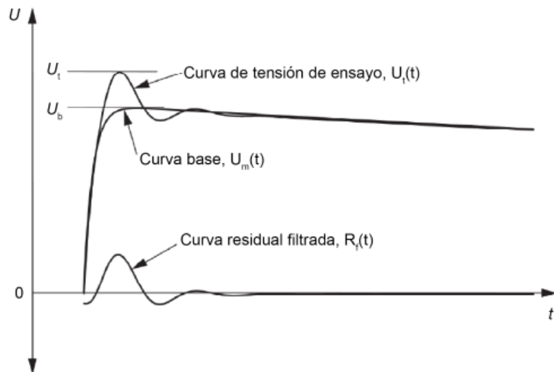
Figura 2.4: Curva tensión de ensayo (suma de curva base y curva residual filtrada). Fuente: [4]. Traducción propia.
