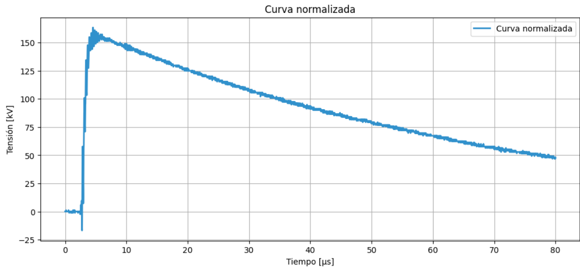
Figura 8.4: Normalización de polaridad. Fuente: Propia.
