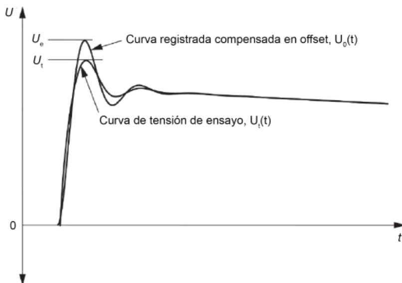
Figura 2.5: Curva tensión de ensayo y curva registrada. Fuente: [4]. Traducción propia.
