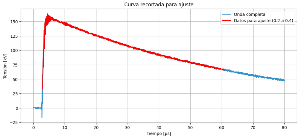
Figura 8.5: Segmentación de datos. Fuente: Propia.
