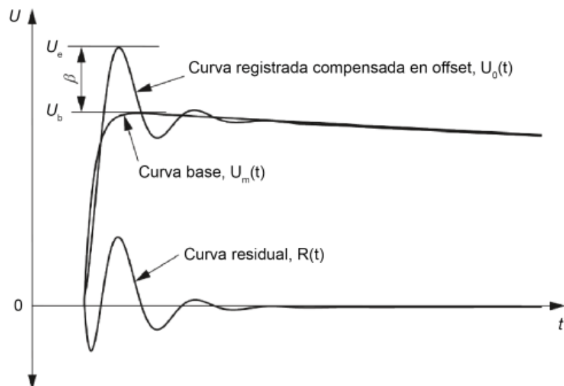
Figura 2.2: Curva registrada con sobreimpulso, curva base y curva residual. Fuente: [4]. Traducción propia.
