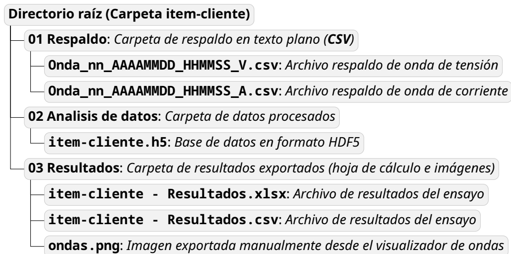
Figura 7.10: Estructura de directorio de archivos. Fuente: Propia.
