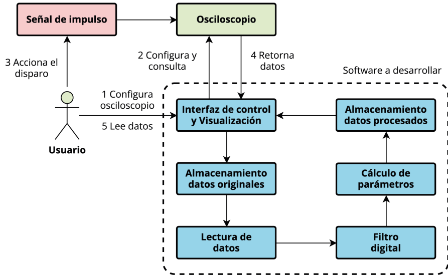
Figura 1.2: Diagrama de solución propuesta. Fuente: Propia.
