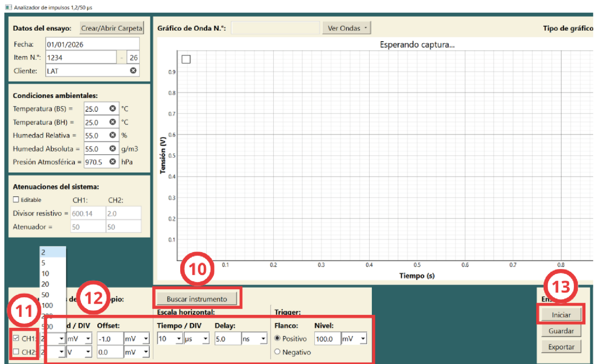
Figura 7.26: Configuración del osciloscopio. Fuente: Propia.
