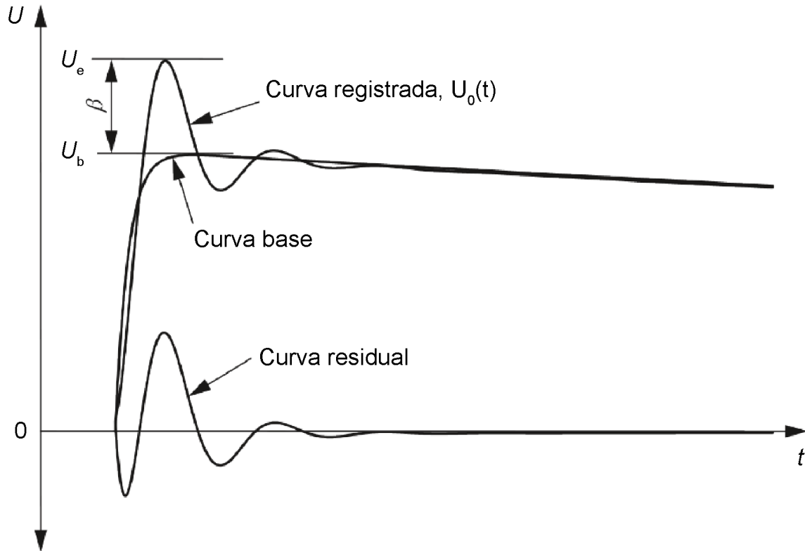
Figura 2.2: Curva registrada con sobreimpulso, curva base y curva residual.
