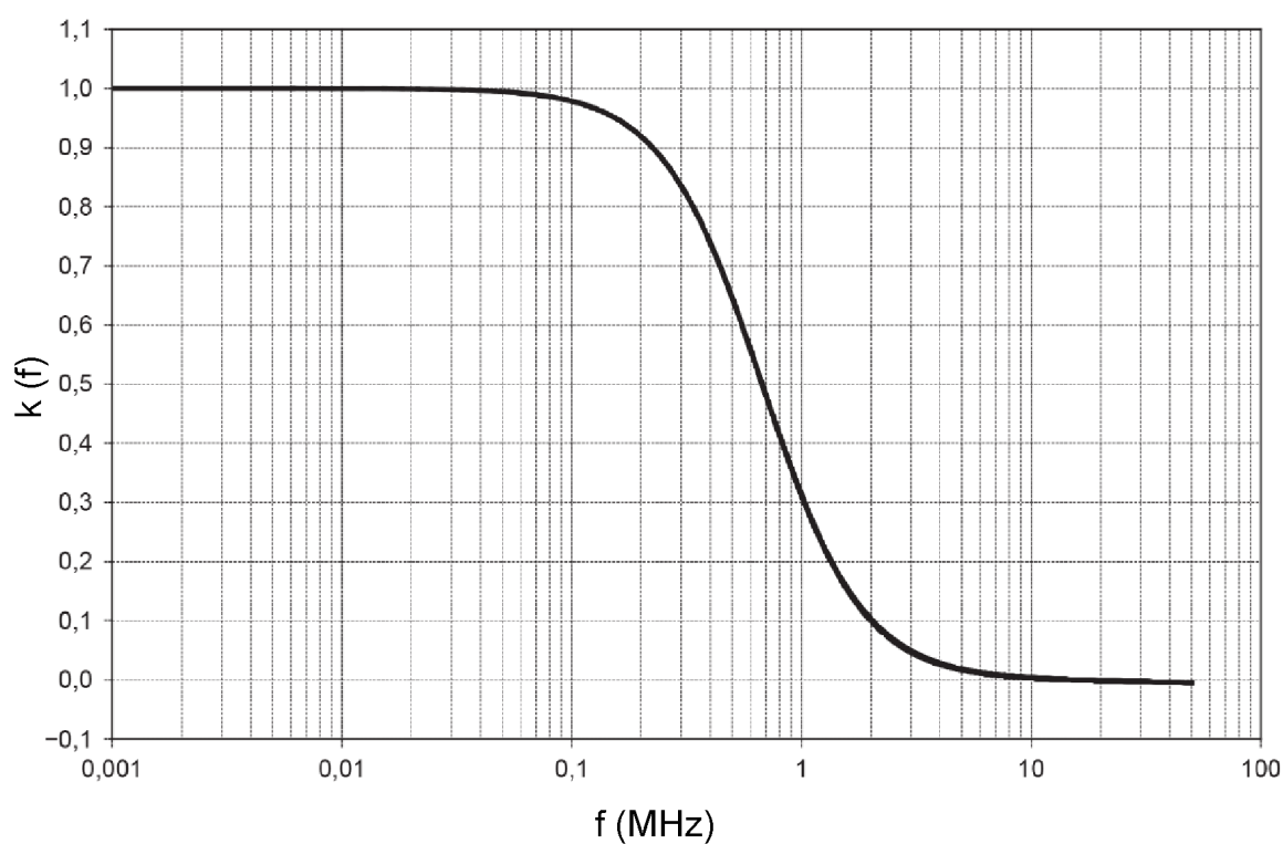
Figura 2.3: Función tensión de ensayo.
