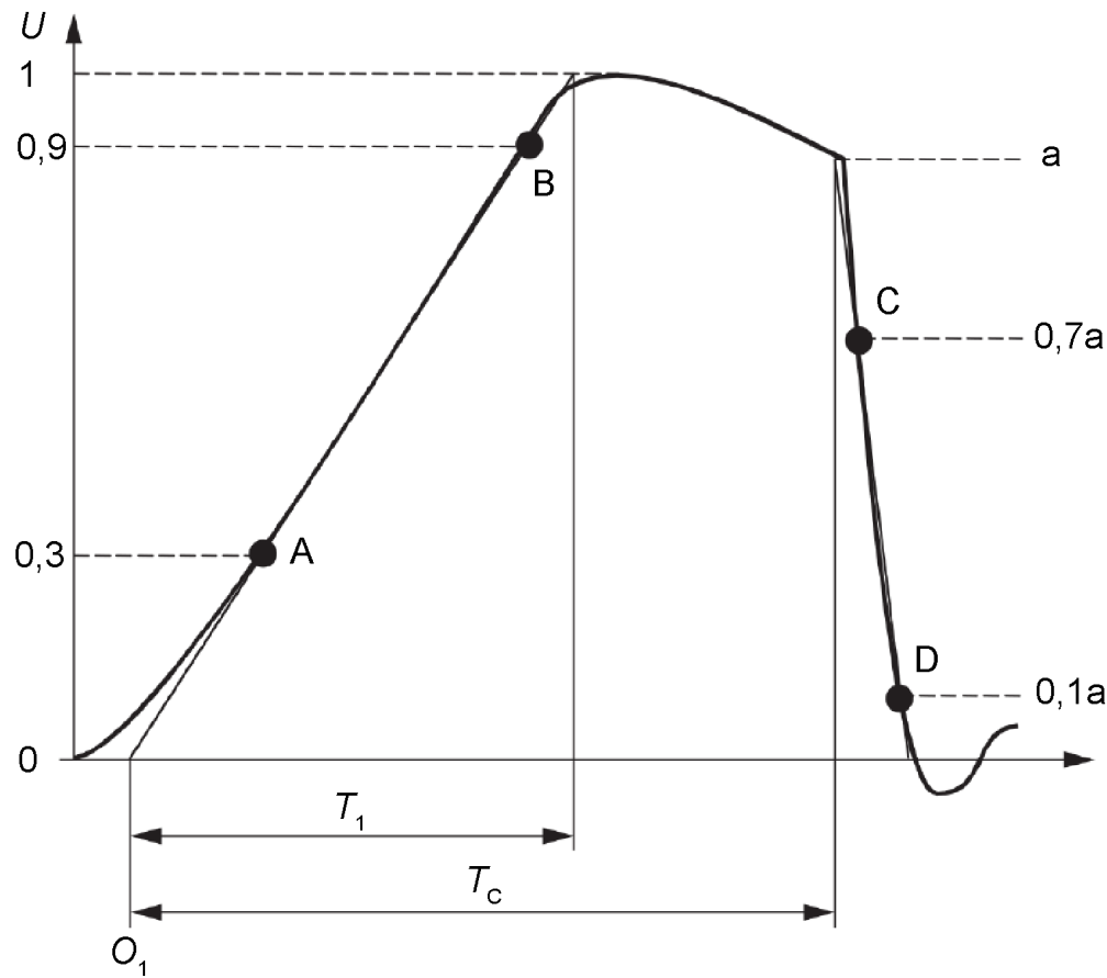
Figura 2.7: Impulso de tensión tipo rayo cortado en la cola.
