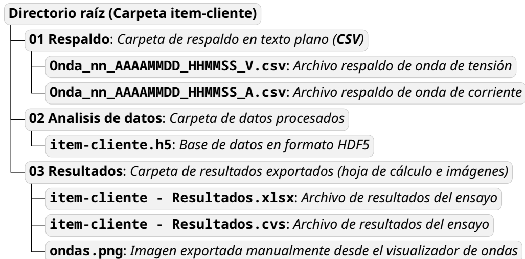
Figura 6.1: Estructura de directorio de archivos.
