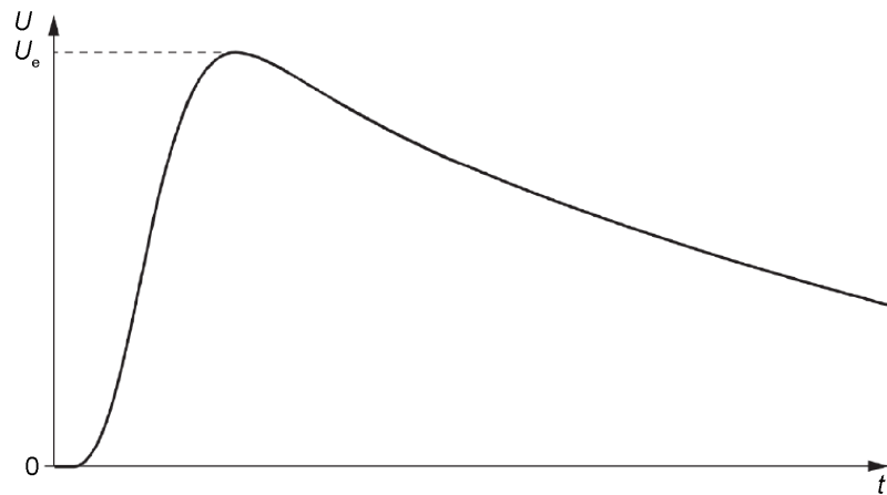
Figura 2.1: Impulso de tensión tipo rayo pleno. Fuente: [4]. Traducción propia.
