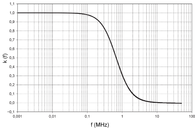
Figura 2.3: Función tensión de ensayo. Fuente: [4]. Traducción propia.
