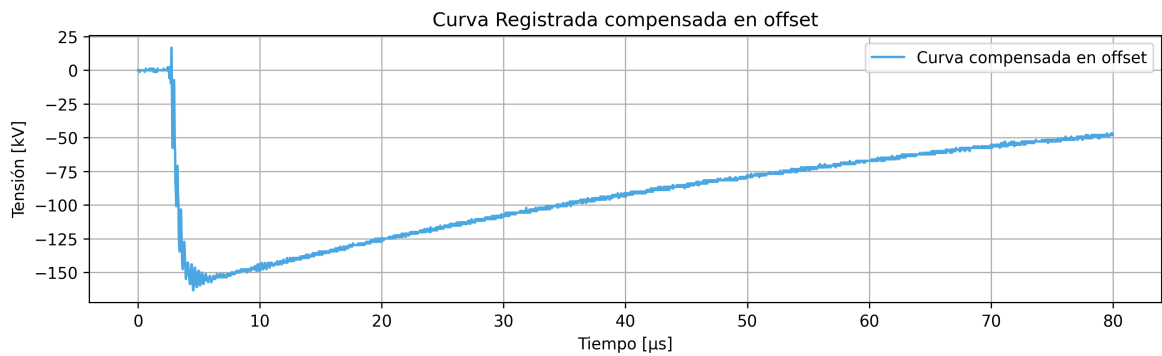
Figura 8.3: Fase I (Acondicionamiento): Curva resultante tras la sustracción del nivel de continua V_{\text{offset}} calculado a partir de las muestras pre-disparo.
