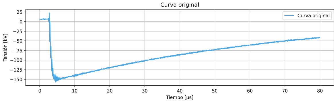
Figura 8.2: Adquisición de datos: Señal discreta bruta U_e[n] adquirida por el instrumento, presentando ruido electromagnético de alta frecuencia y nivel de continua previo al disparo.
