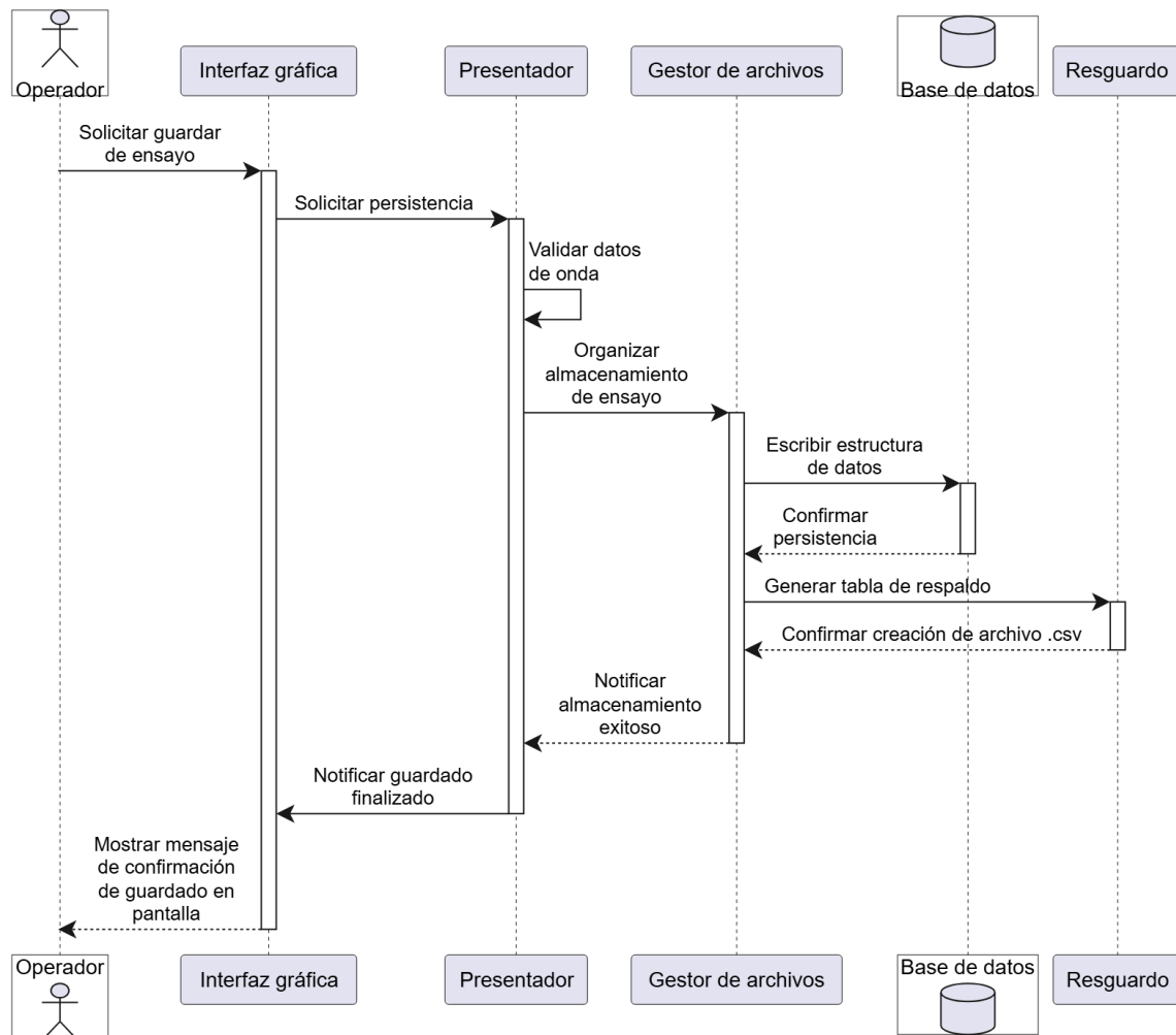
Figura 7.8: Diagrama de secuencia del guardado de información. Fuente: Propia.
