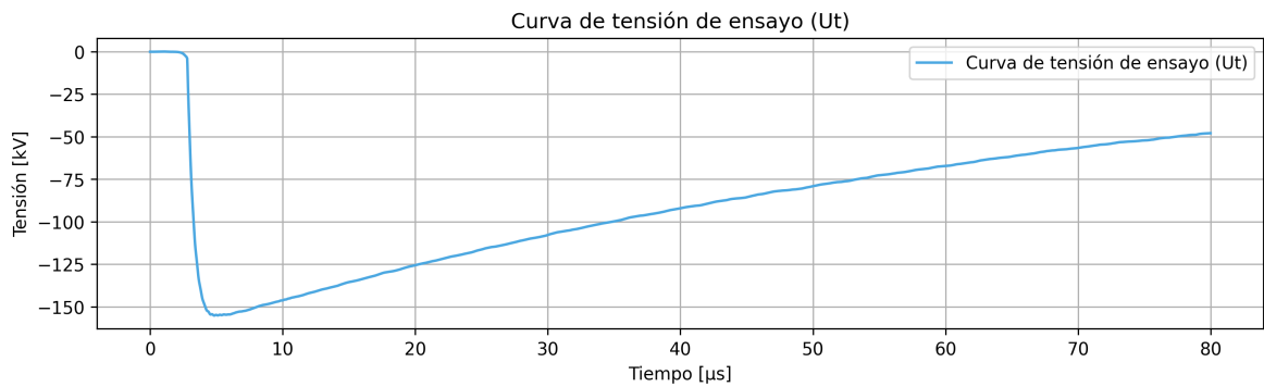
Figura 8.9: Fase III (Síntesis): Curva de tensión de ensayo U_t[n] , producto de la suma-toria entre la curva base y la curva residual filtrada (ecuación 7.23).
