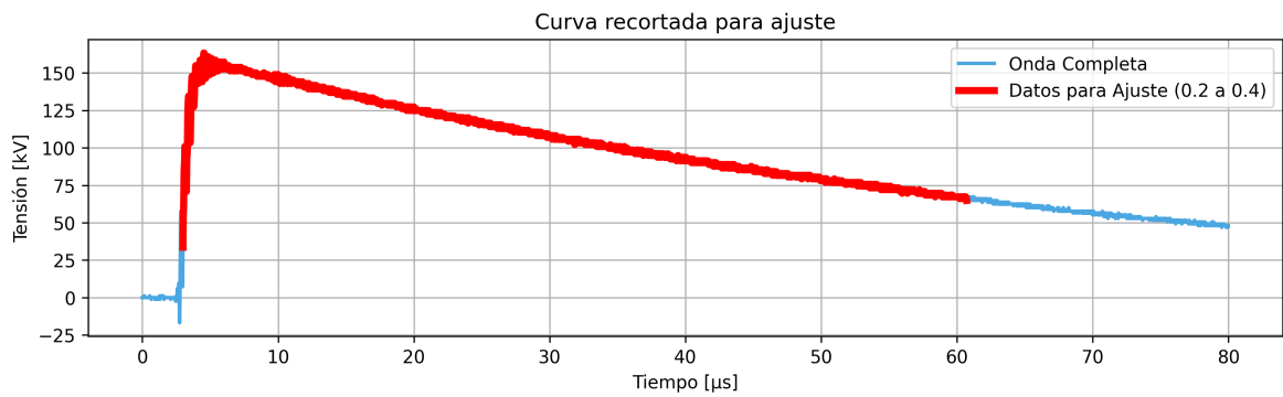
Figura 8.5: Fase II (Segmentación): Delimitación de la ventana de datos útil (comprendida entre el 20 % del frente y el 40 % de la cola) para la regresión no lineal con el algoritmo de Levenberg-Marquardt [2].
