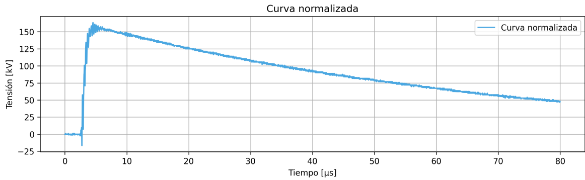
Figura 8.4: Fase I (Normalización): Curva con polaridad normalizada hacia el semi-plano positivo.
