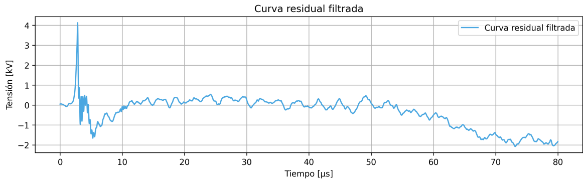
Figura 8.8: Fase III (Filtrado): Curva residual filtrada R_f[n] tras aplicar el filtro digital IIR de fase cero bidireccional (con la característica de la ecuación 2.3), que mitiga la distorsión morfológica.
