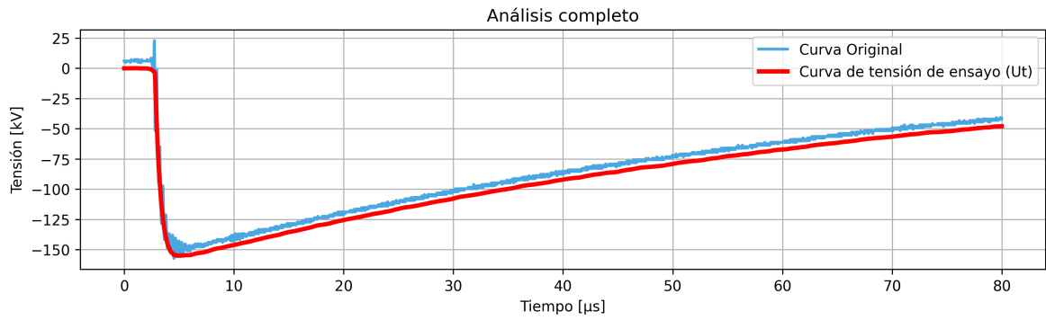
Figura 8.10: Resultado Final: Comparativa superpuesta entre la curva de tensión de ensayo procesada frente a la señal original bruta, evidenciando la eliminación de perturbaciones, lista para la extracción de sus parámetros U_t , T_1 , T_2 y OS%.
