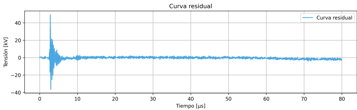
Figura 8.7: Fase III (Convergencia): Curva residual R[n] obtenida por la diferencia algebraica entre la señal registrada y la curva base (ecuación 7.22), aislando las oscilaciones y el ruido.
