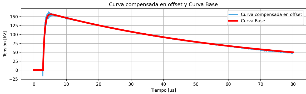
Figura 8.6: Fase II (Ajuste de curva): Curva base U_b[n] sintetizada sobre una función doble exponencial (ecuación 4.1), superpuesta a la señal registrada.
