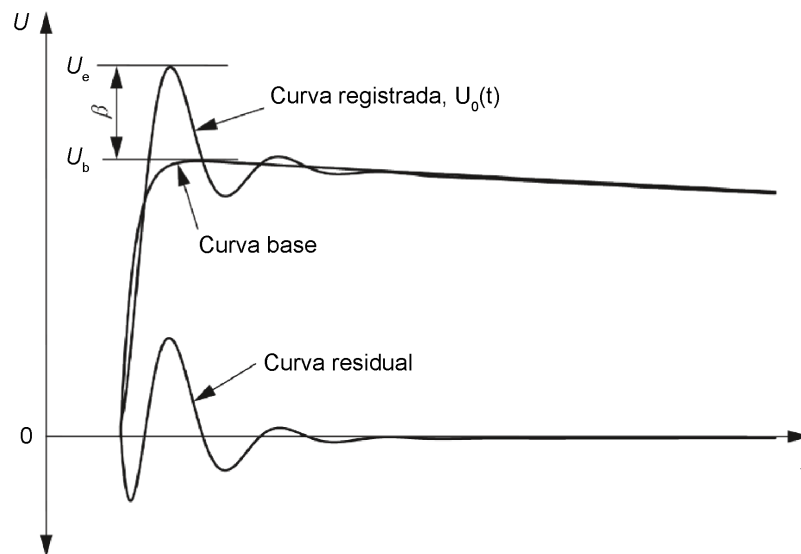
Figura 2.2: Curva registrada con sobreimpulso, curva base y curva residual. Fuente: [4]. Traducción propia.
