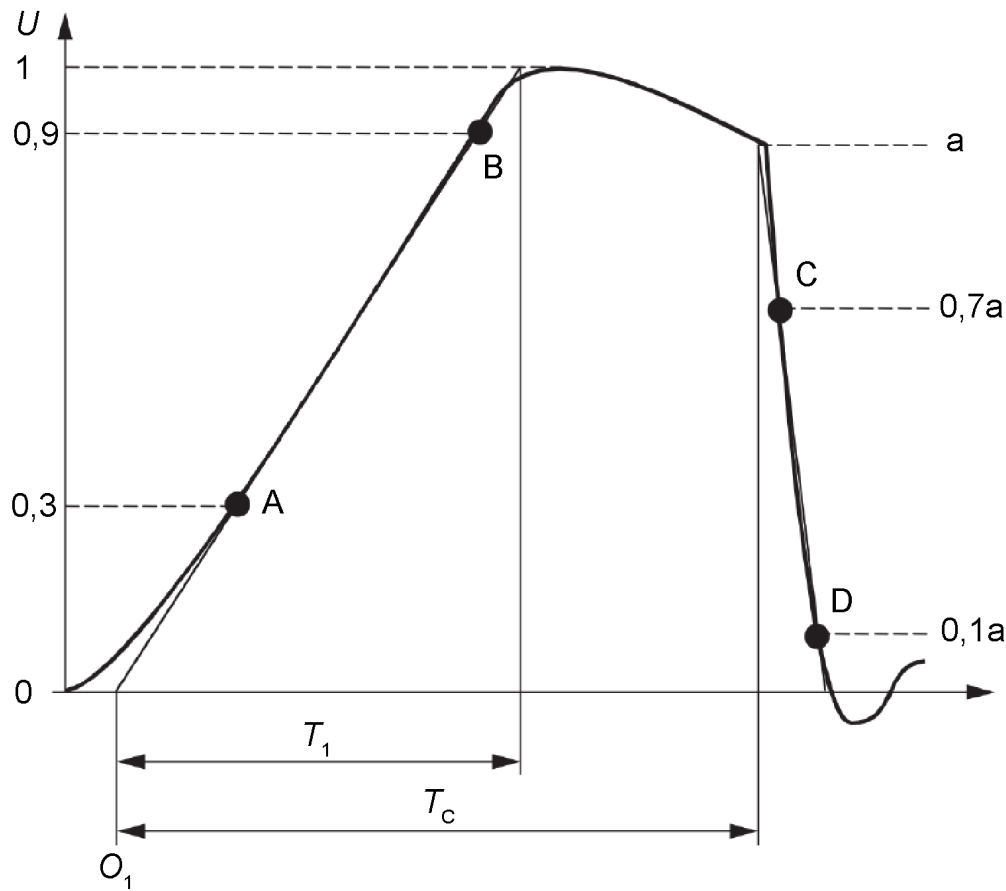
Figura 1.7: Impulso de tensión tipo rayo cortado en la cola.
