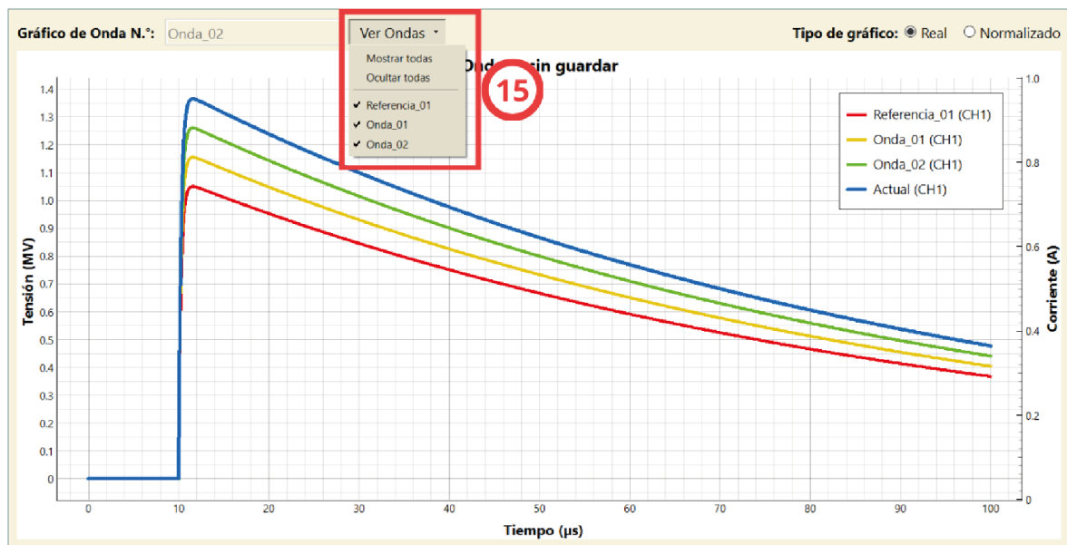
Figura 5.20: Historial de impulsos guardados.
