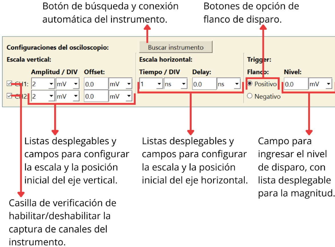
Figura 5.9: Bloque de Control del instrumento.
