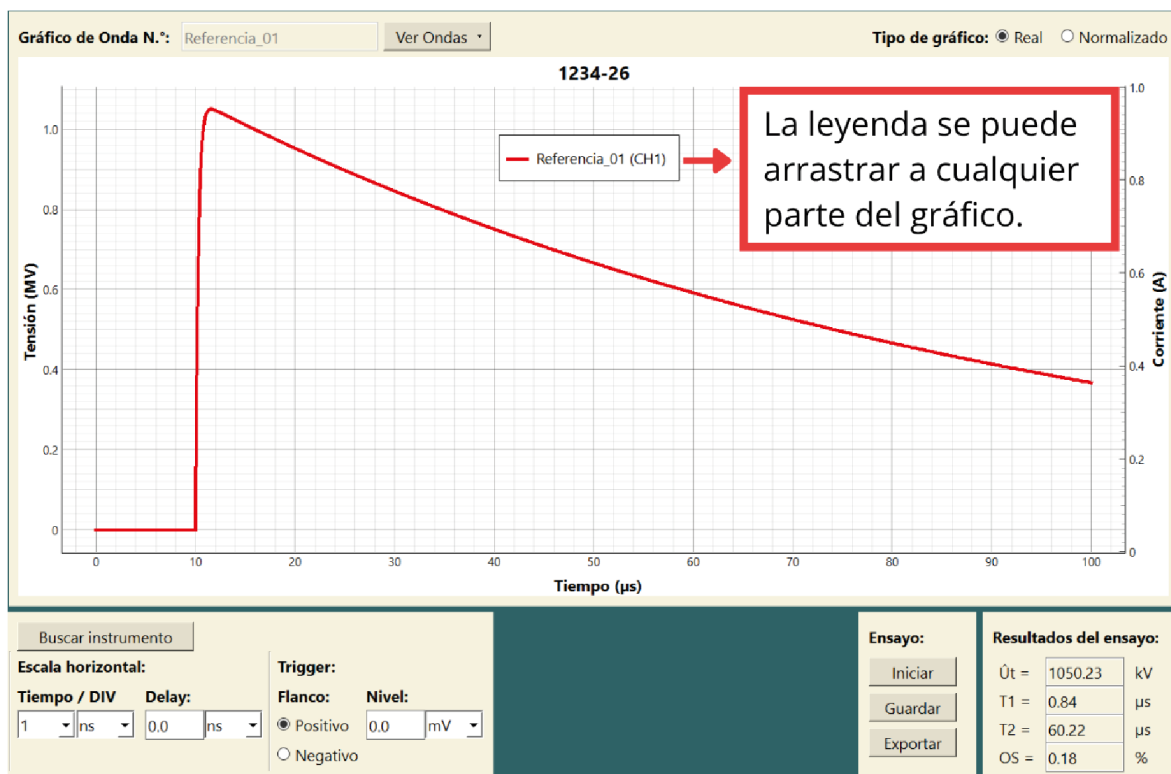
Figura 5.19: Ejemplo de onda guardada.
