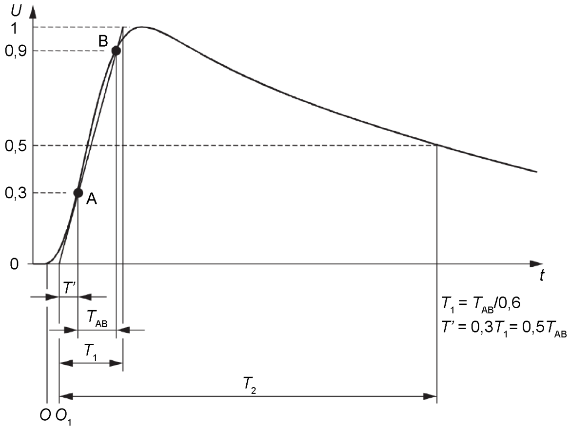
Figura 1.6: Parámetros de tiempo del impulso de tensión tipo rayo pleno.
