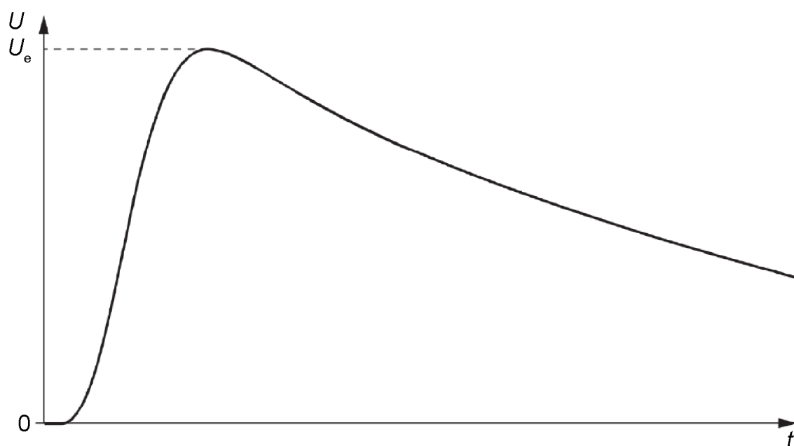
Figura 1.1: Impulso de tensión tipo rayo pleno.
