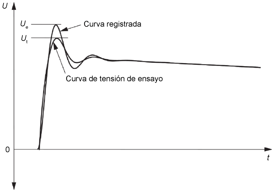
Figura 1.5: Curva tensión de ensayo y curva registrada.
