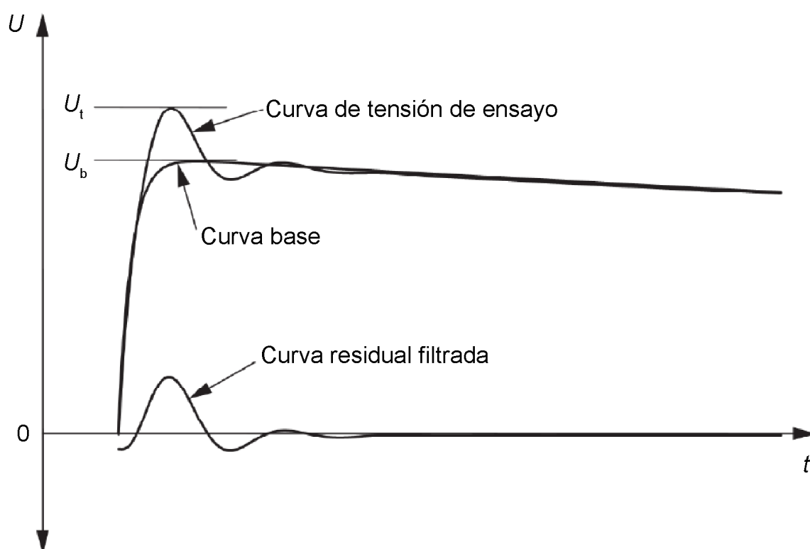
Figura 1.4: Curva tensión de ensayo (suma de curva base y curva residual filtrada).
