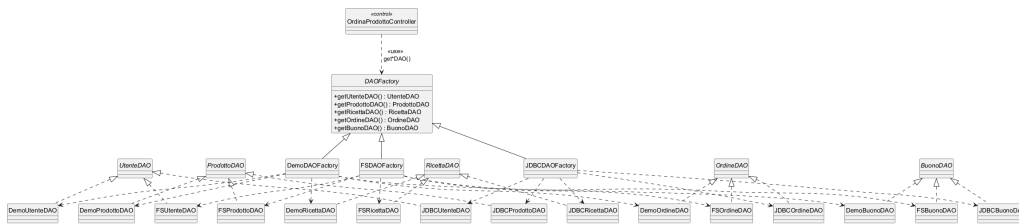
Figura 3.2: Design-level: Abstract Factory della persistenza (DAOFactory + concrete factory Demo/FS/JDBC e interfacce DAO).
