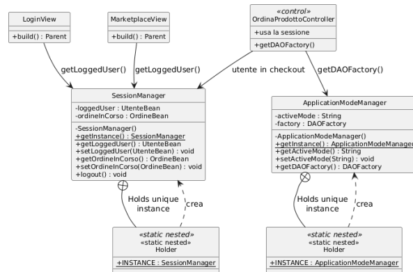
Figura 3.5: Design-level: Singleton della sessione e della modalità applicativa.
