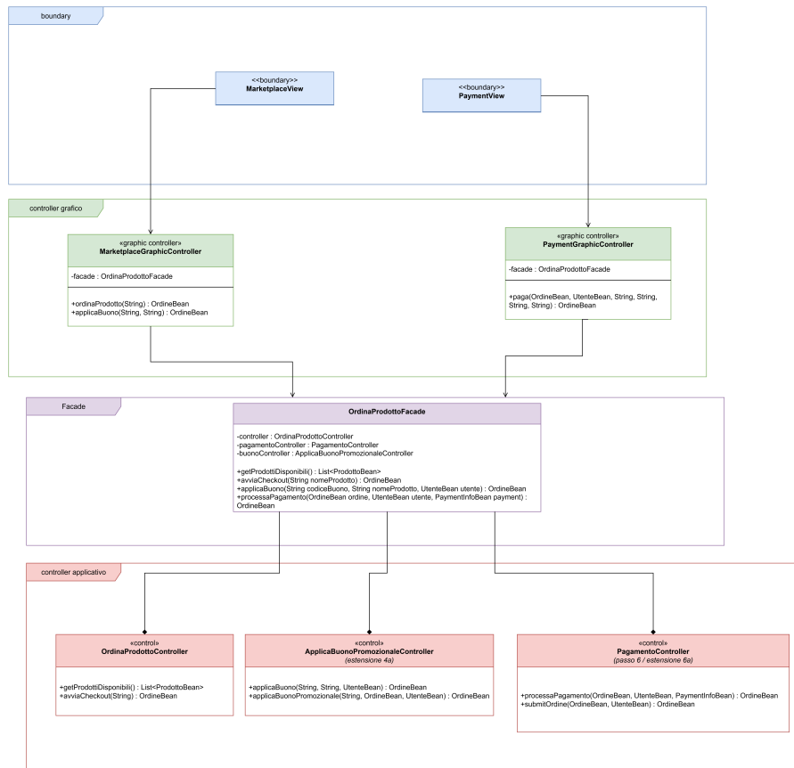
Figura 3.5: Facade del checkout di UC-04.
