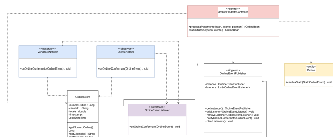
Figura 3.3: Observer della conferma dell'ordine: publisher singleton e DTO.
