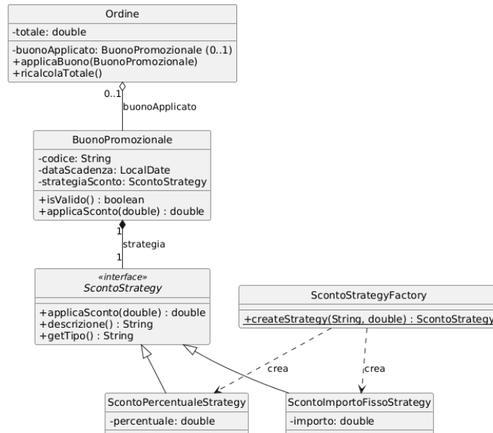
Figura 3.3: Design-level: sotto-sistema del buono promozionale (Context Ordine, Strategy sconto e factory).
