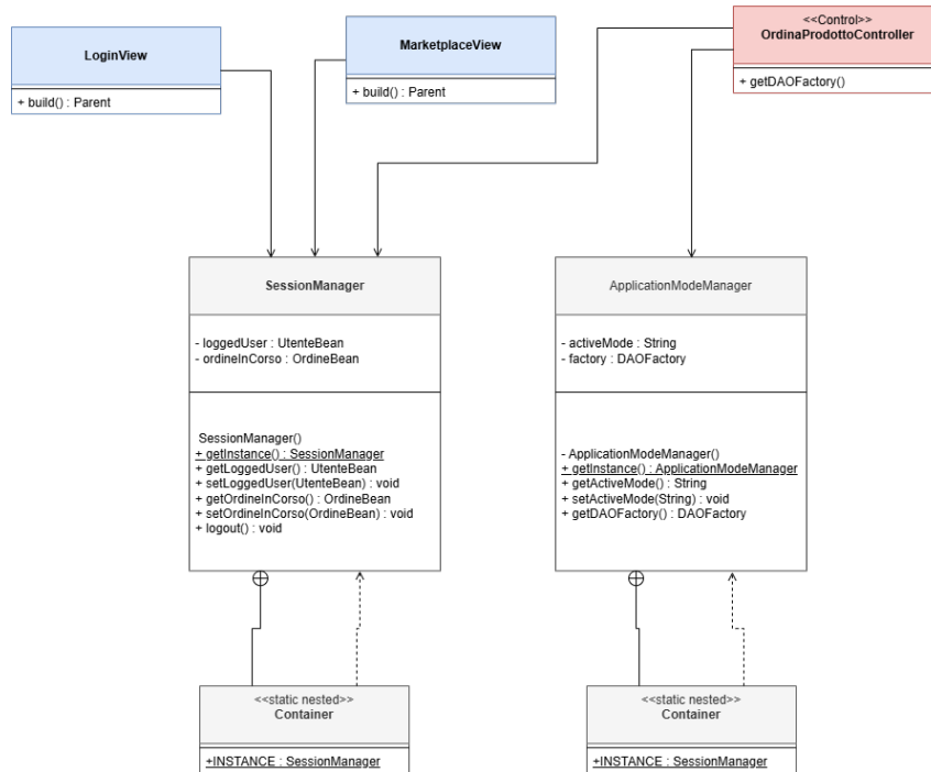
Figura 3.5: Design-level: Singleton della sessione e della modalità applicativa.
