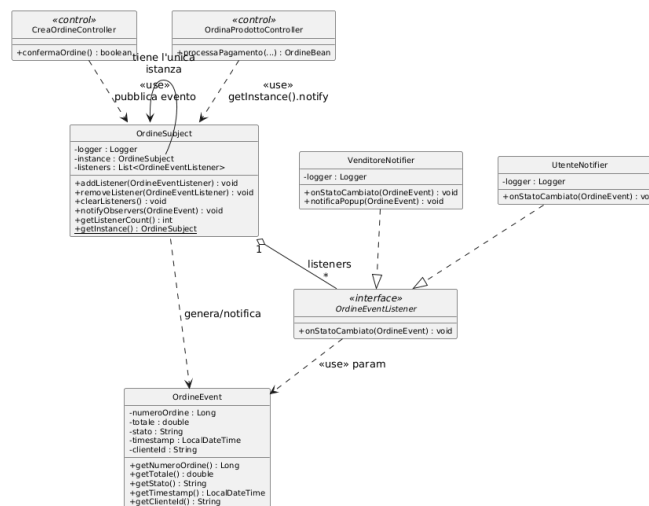
Figura 3.4: Design-level: sistema di notifica asincrona (Observer Subject/listener/notifier).
