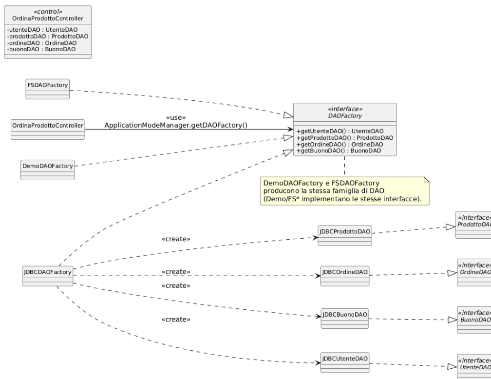
Figura 3.2: Design-level: Abstract Factory della persistenza (DAOFactory + concrete factory Demo/FS/JDBC e interfacce DAO).
