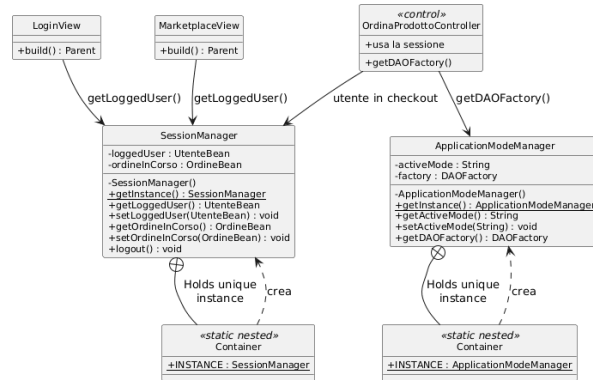
Figura 3.5: Design-level: Singleton della sessione e della modalità applicativa.
