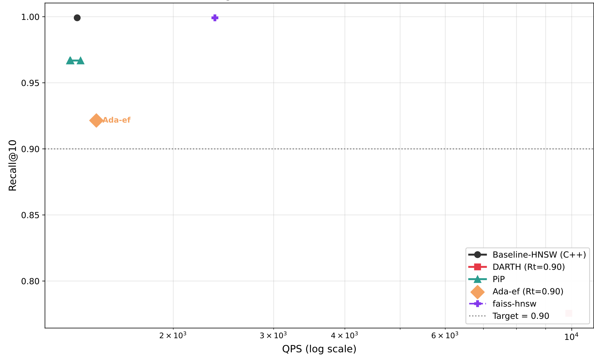
Recall@10 vs QPS — sift128 (M=16, efC=200)
