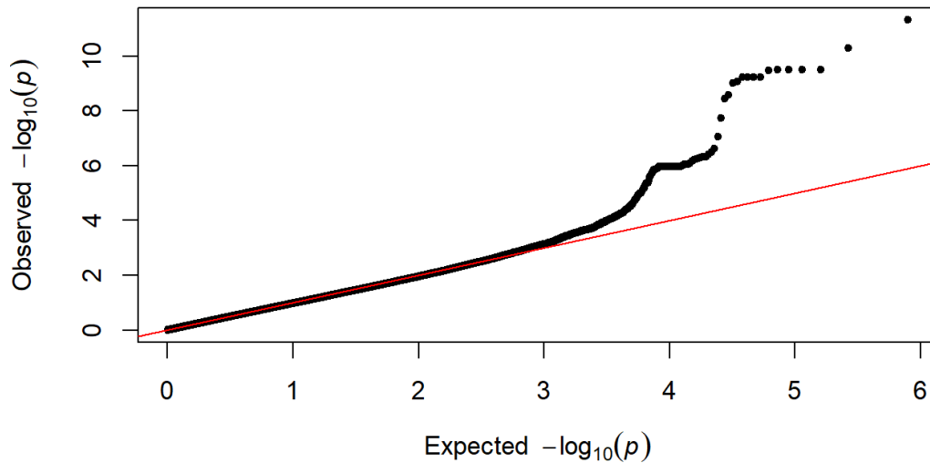
FIGURE 11 – QQ plot pour le site viral 1276
