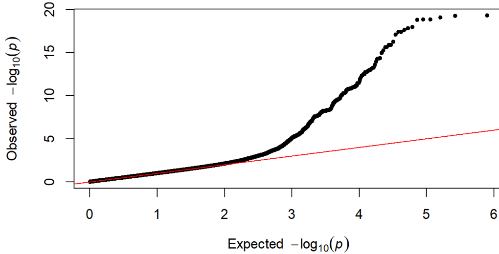
FIGURE 9 – QQ plot pour le site viral 1450
