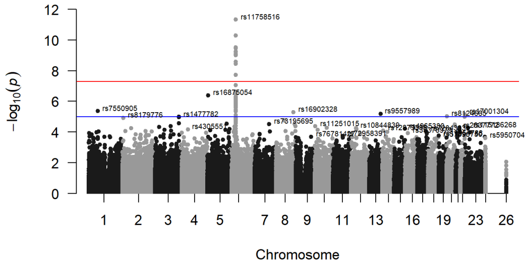
FIGURE 10 – Manhattan plot pour le site viral 1276
