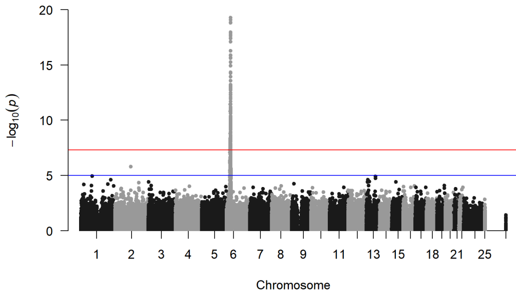
FIGURE 8 – Manhattan plot pour le site viral 1450
