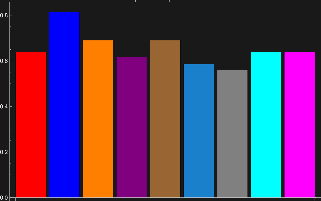
Норма L_\infty при t = 3.60
