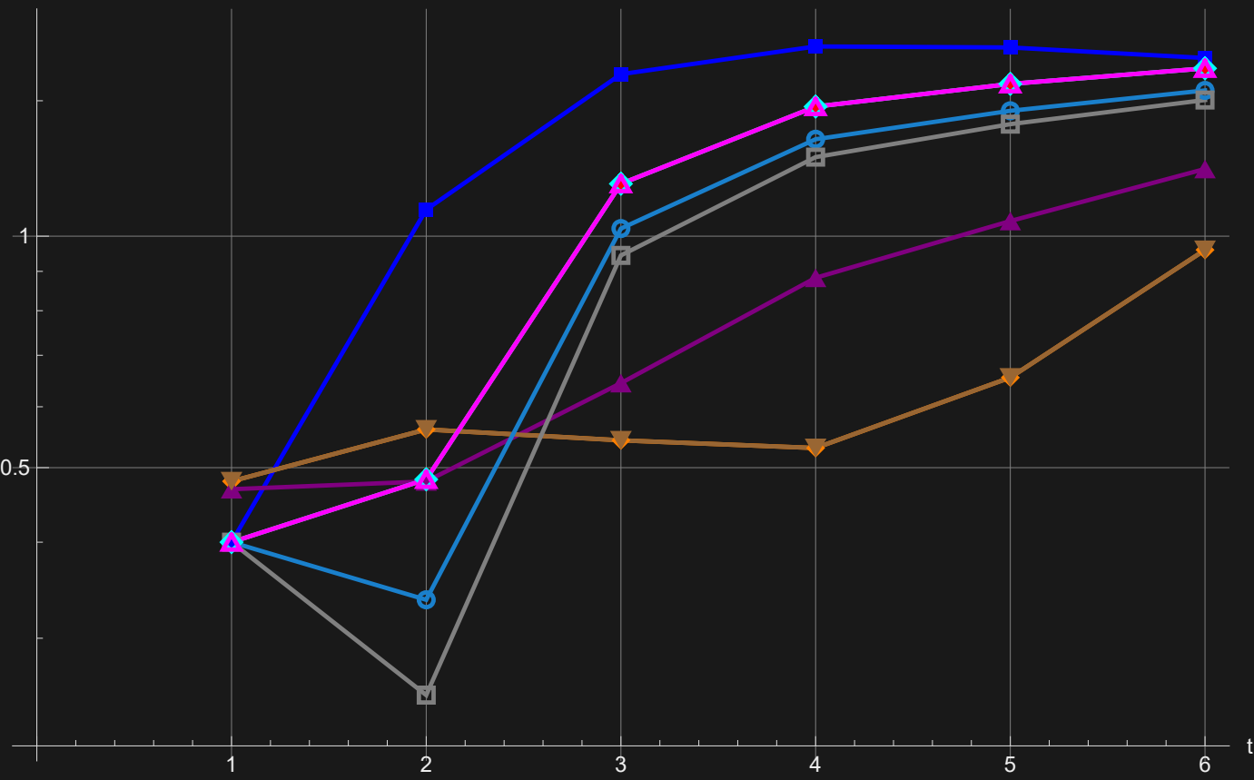
Норма L1 (логарифмическая шкала)
