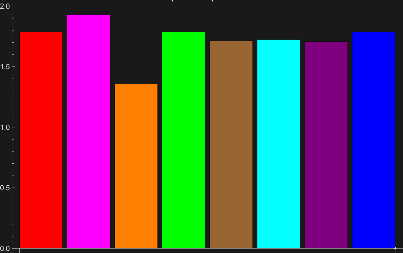
Норма L2 при t = 250
