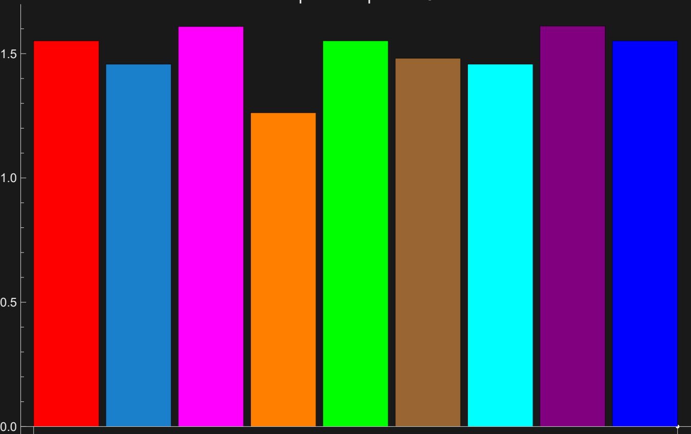
Норма L1 при t = 40
