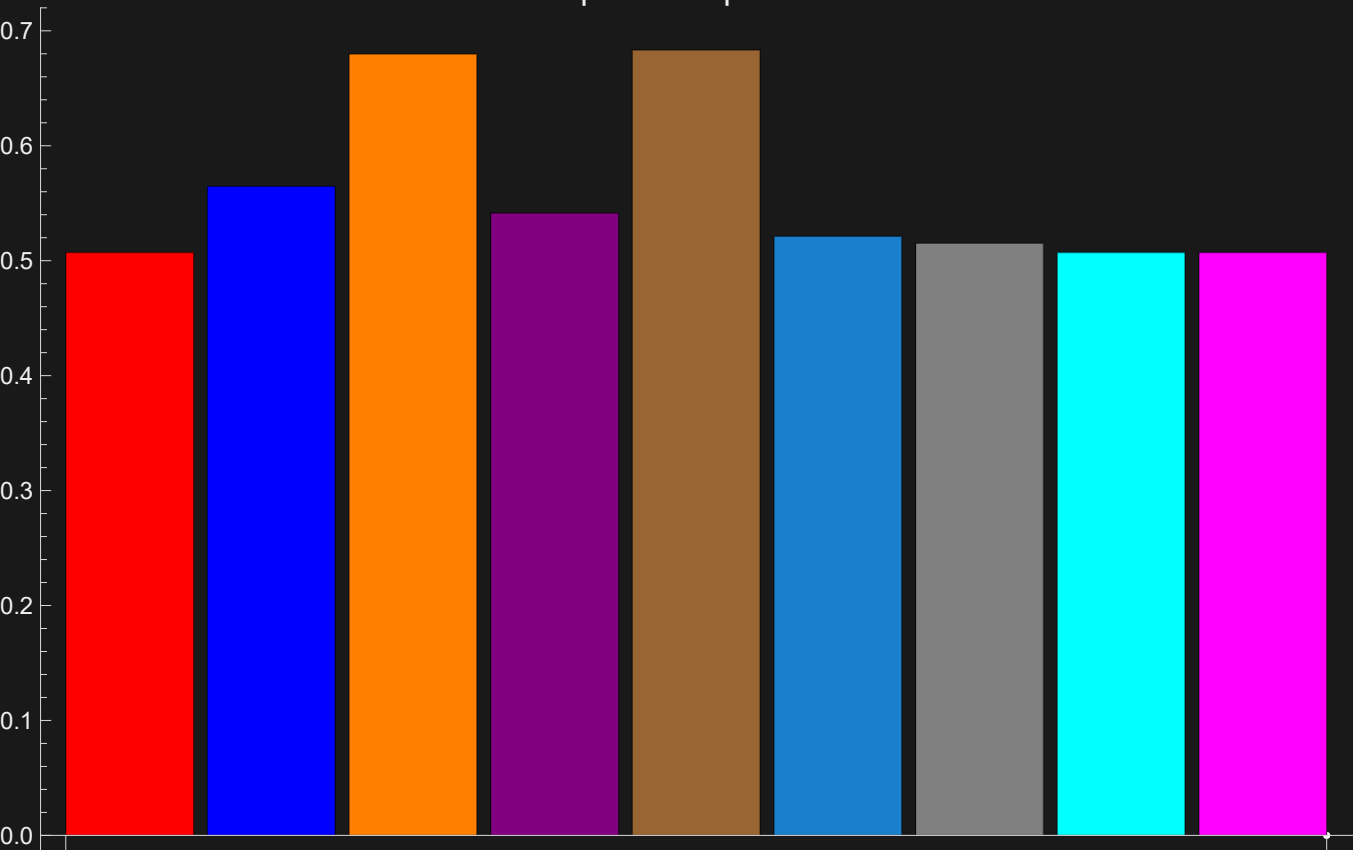
Норма L_\infty при t = 16
