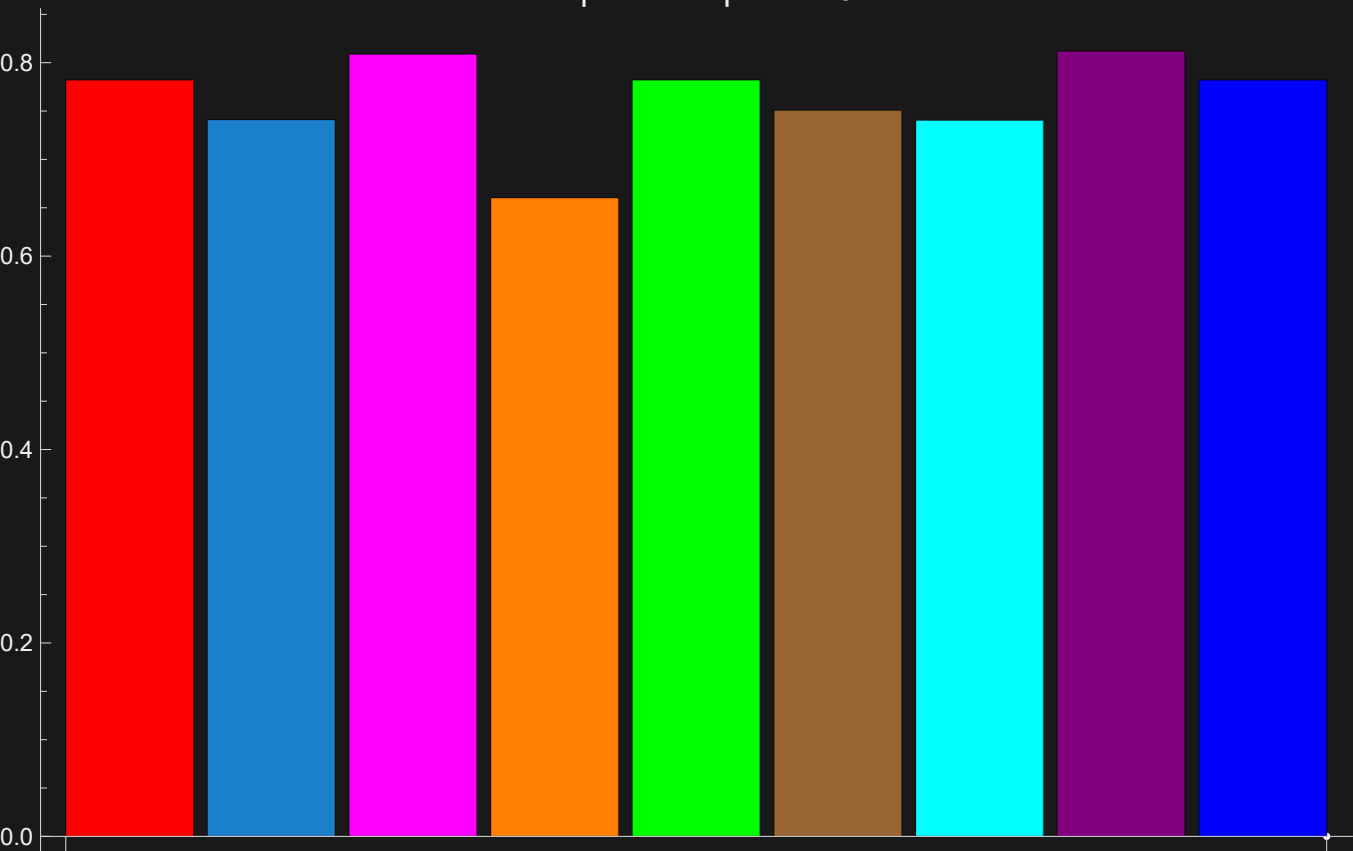
Норма L_\infty при t = 40
